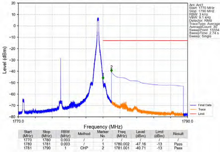
Band66_10MHz_QPSK_HCH_1775MHz_RB_1_49_NTNV
