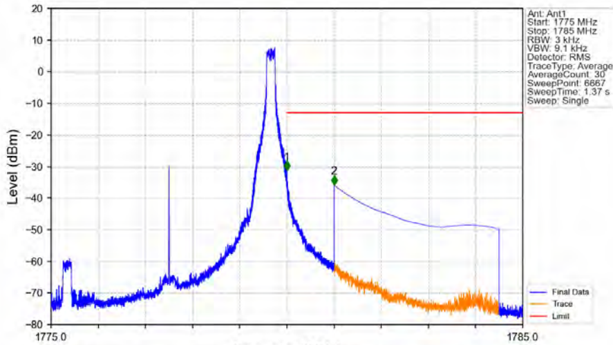
Band66_5MHz_QPSK_HCH_1777.5MHz_RB_1_24_NTNV
