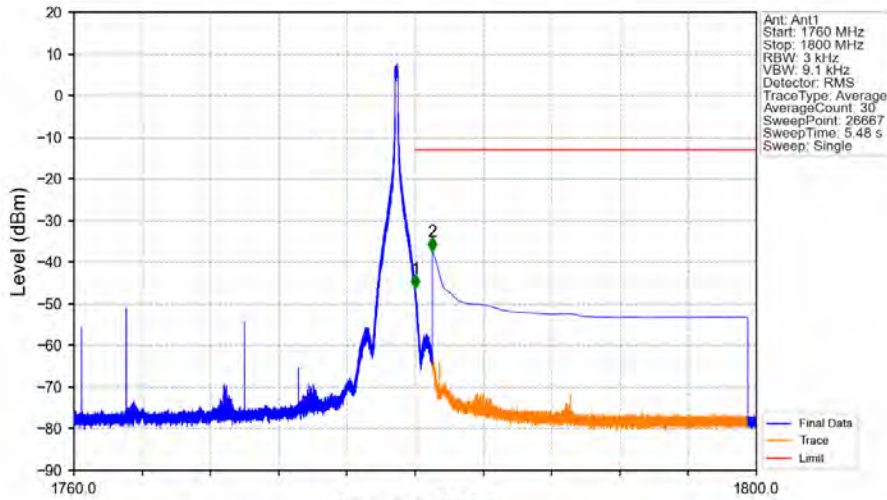
Band66_20MHz_QPSK_HCH_1770MHz_RB_1_99_NTNV
