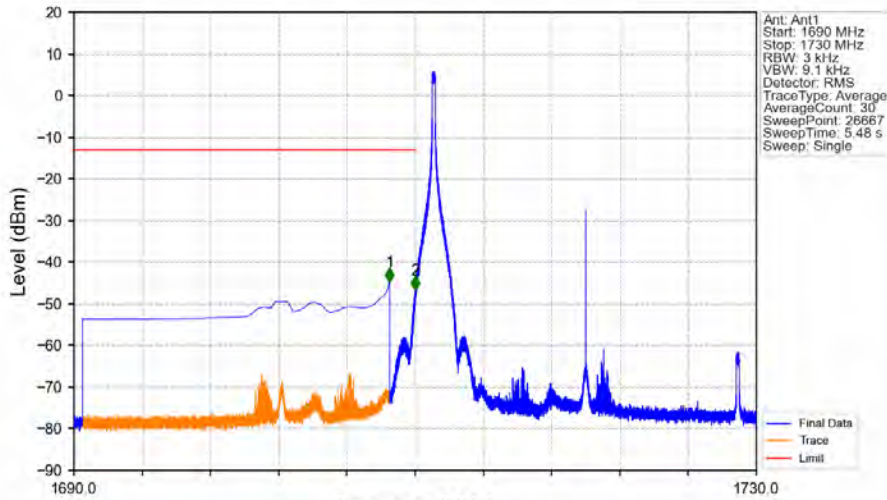
Band66_20MHz_16QAM_LCH_1720MHz_RB_1_0_NTNV
