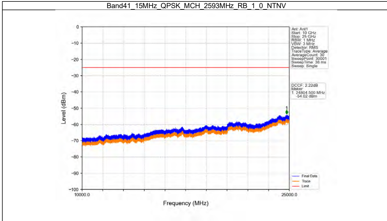
Band41_15MHz_QPSK_MCH_2593MHz_RB_1_0_NTNV
