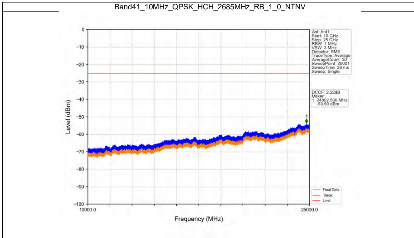
Band41_10MHz_QPSK_HCH_2685MHz_RB_1_0_NTNV
