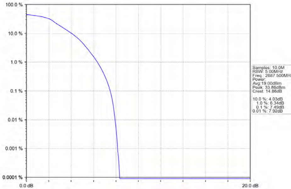
Band41_5MHz_QPSK_HCH_2687.5MHz_RB_25_0_NTNV
