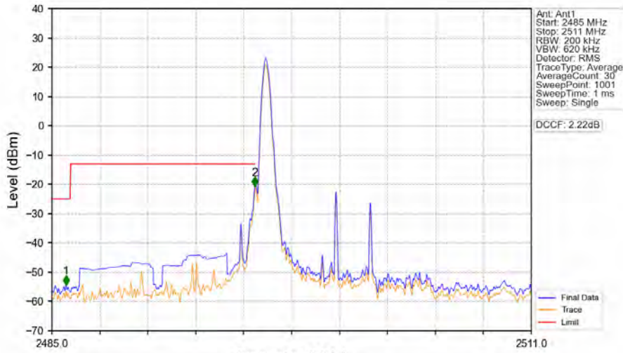
Band41_10MHz_16QAM_LCH_2501MHz_RB_1_0_NTNV
