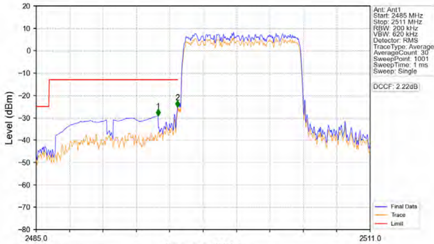
Band41_10MHz_QPSK_LCH_2501MHz_RB_50_0_NTNV
