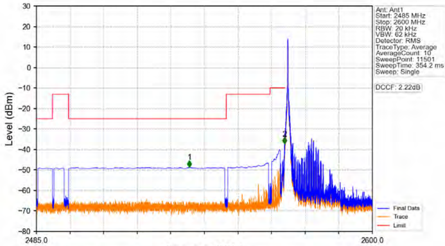
Band38_20MHz_16QAM_LCH_2580MHz_RB_1_0_NTNV
