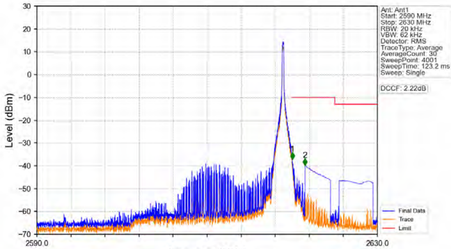
Band38_20MHz_QPSK_HCH_2610MHz_RB_1_99_NTNV
