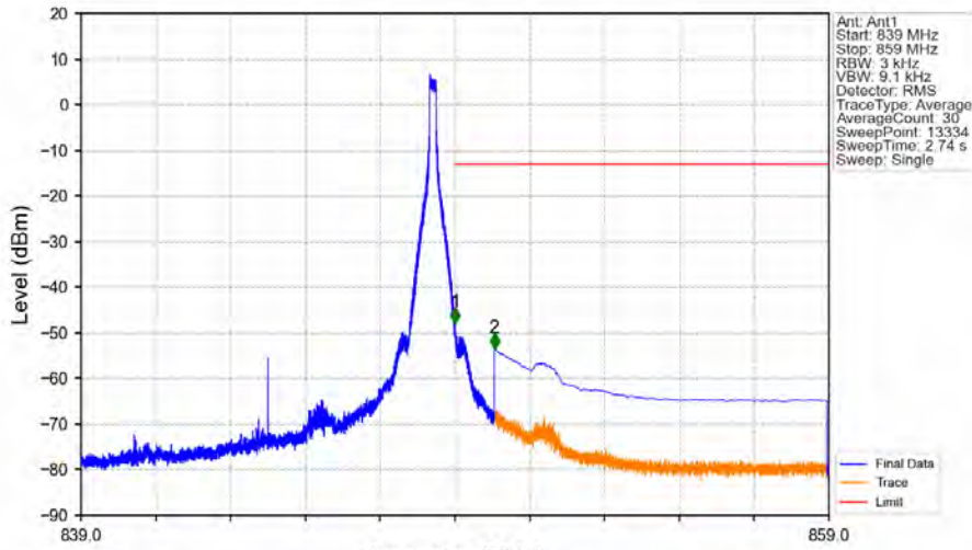
Band26b_10MHz_QPSK_HCH_844MHz_RB_1_49_NTNV
