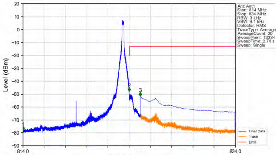
Band26a_10MHz_QPSK_HCH_819MHz_RB_1_49_NTNV
