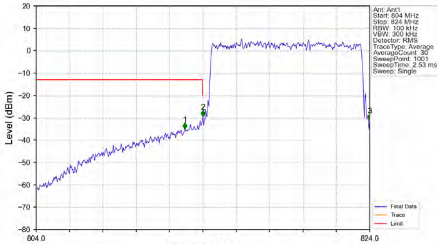
Band26a_10MHz_QPSK_LCH_819MHz_RB_50_0_NTNV
