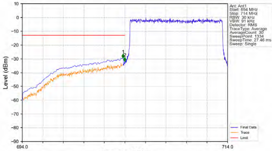
Band17_10MHz_QPSK_LCH_709MHz_RB_50_0_NTNV
