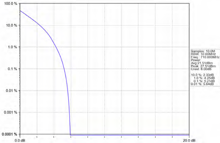
Band17_10MHz_QPSK_MCH_710MHz_RB_50_0_NTNV
