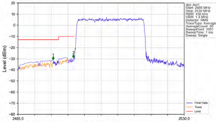
Band7_20MHz_QPSK_LCH_2510MHz_RB_100_0_NTNV
