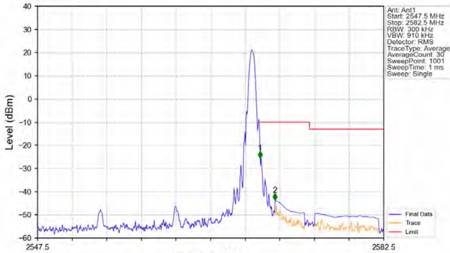
Band7_15MHz_QPSK_HCH_2562.5MHz_RB_1_74_NTNV
