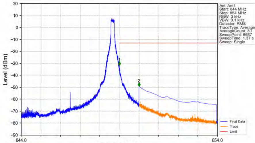
Band5_5MHz_QPSK_HCH_846.5MHz_RB_1_24_NTNV
