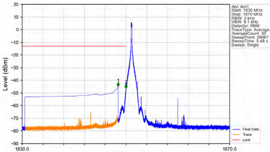
Band2_20MHz_64QAM_LCH_1860MHz_RB_1_0_NTNV
