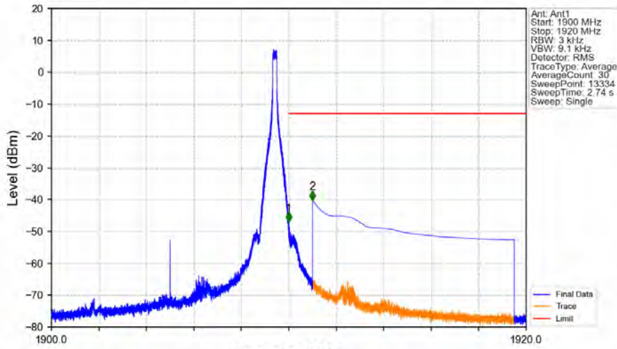
Band2_10MHz_QPSK_HCH_1905MHz_RB_1_49_NTV
