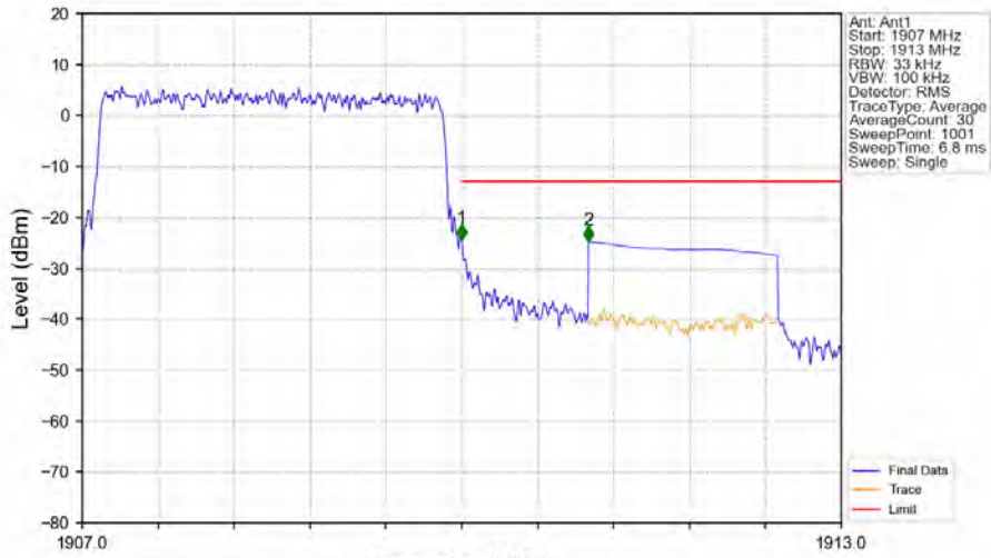
Band2_3MHz_QPSK_HCH_1908.5MHz_RB_15_0_NTNV
