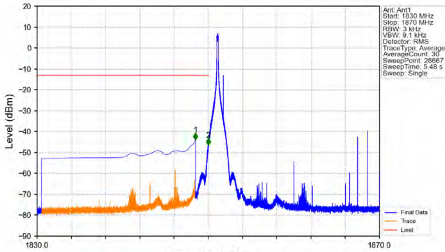
Band2_20MHz_16QAM_LCH_1860MHz_RB_1_0_NTNV
