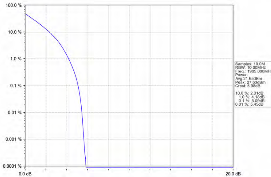
Band2_10MHz_QPSK_HCH_1905MHz_RB_50_0_NTNV
