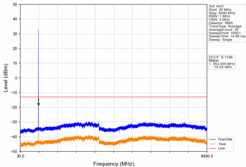
GSM850_GSM_HCH_848.8MHz_GSM_NTNV
