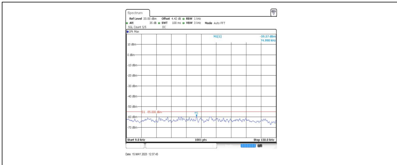
7-7-20MHz-20MHz-QPSK-QPSK-21001-21199-1RB#0-0RB#0-0.009~0.15MHz
