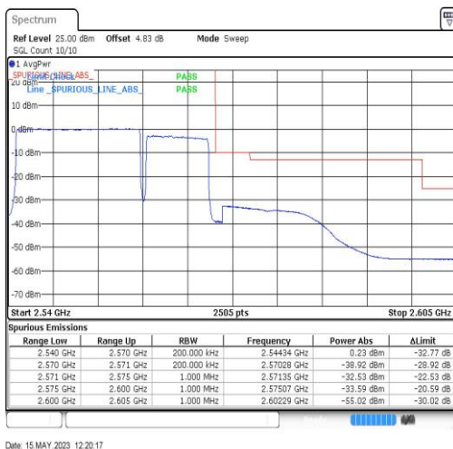
7-7-20MHz-10MHz-QPSK-QPSK-21251-21395-100RB#0-50RB#0
