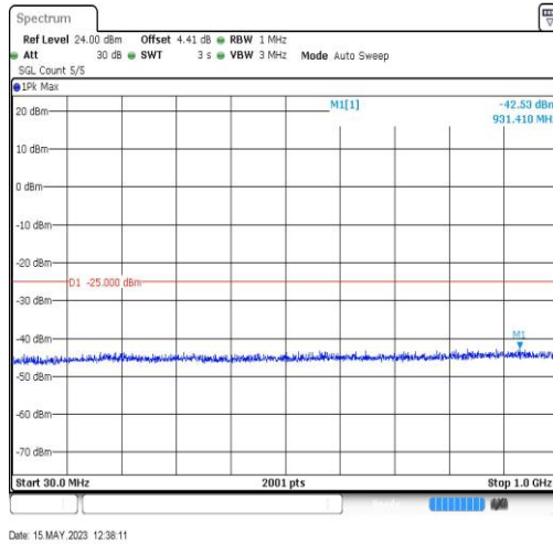
7-7-20MHz-20MHz-QPSK-QPSK-21001-21199-1RB#0-0RB#0-30~1000MHz
