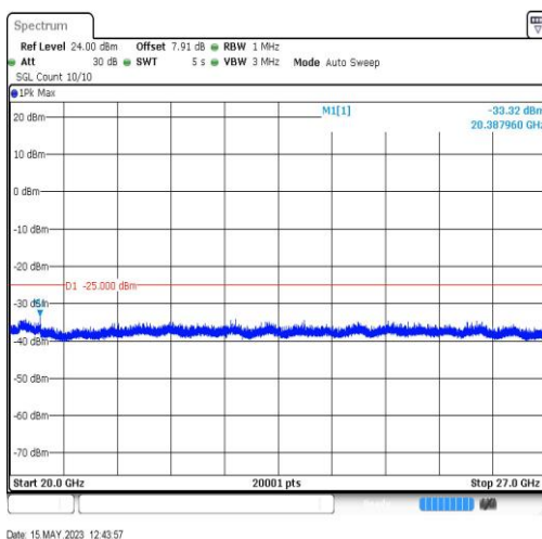
7-7-20MHz-20MHz-QPSK-QPSK-21152-21350-1RB#0-0RB#0-20000~27000MHz
