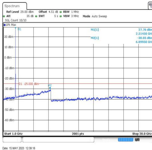
7-7-20MHz-20MHz-QPSK-QPSK-21001-21199-1RB#0-0RB#0-1000~20000MHz
