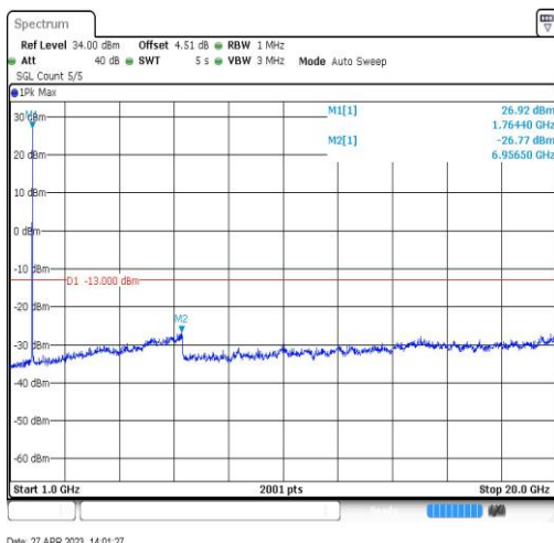
Band66-20MHz-QPSK-132572-1RB#0-Range4:1000~20000MHz
