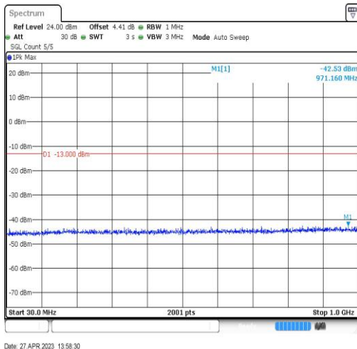
Band66-20MHz-QPSK-132072-1RB#0-Range3:30~1000MHz
