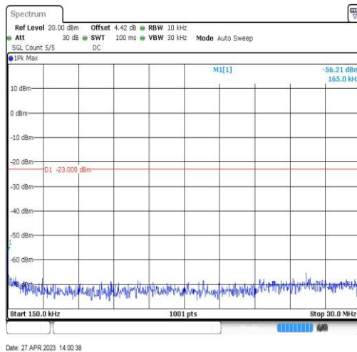
Band66-20MHz-QPSK-132572-1RB#0-Range2:0.15~30MHz
