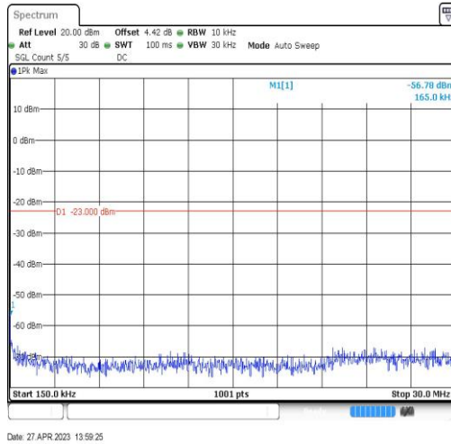
Band66-20MHz-QPSK-132322-1RB#0-Range2:0.15~30MHz
