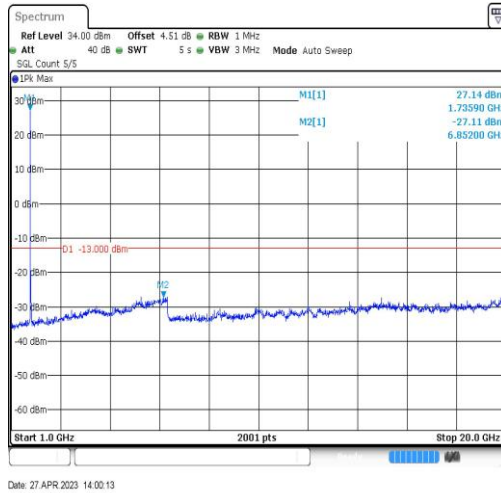
Band66-20MHz-QPSK-132322-1RB#0-Range4:1000~20000MHz
