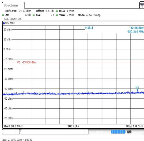
Band66-20MHz-QPSK-132572-1RB#0-Range3:30~1000MHz
