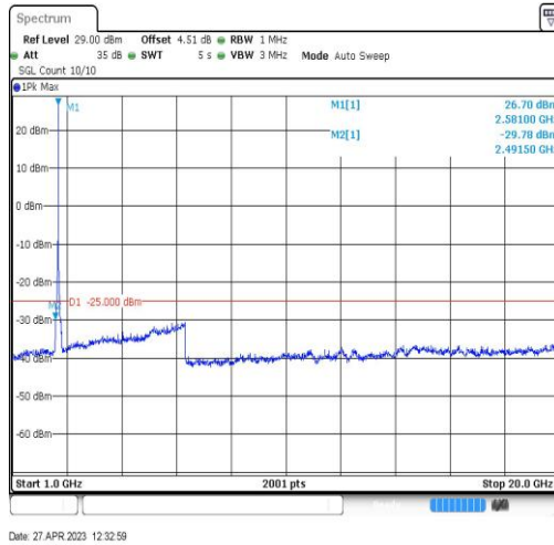
Band41-20MHz-QPSK-40620-1RB#0-Range4:1000~20000MHz
