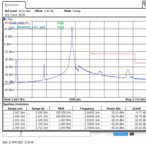
Band41-20MHz-QPSK-41490-1RB#99
