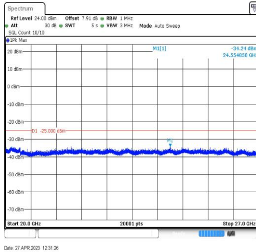
Band41-20MHz-QPSK-39750-1RB#0-Range5:20000~27000MHz
