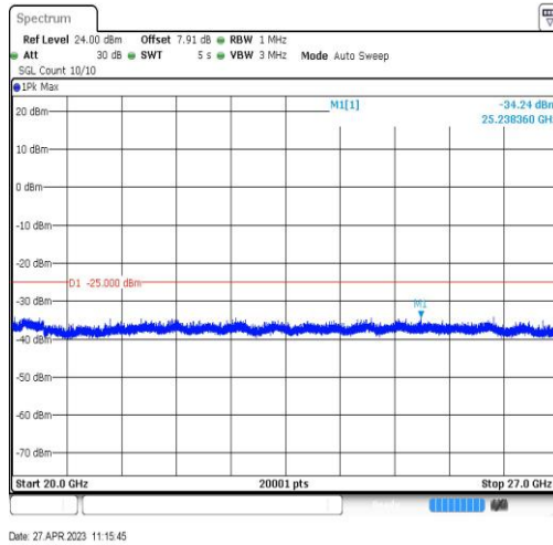
Band38-20MHz-QPSK-38150-1RB#0-Range5:20000~27000MHz
