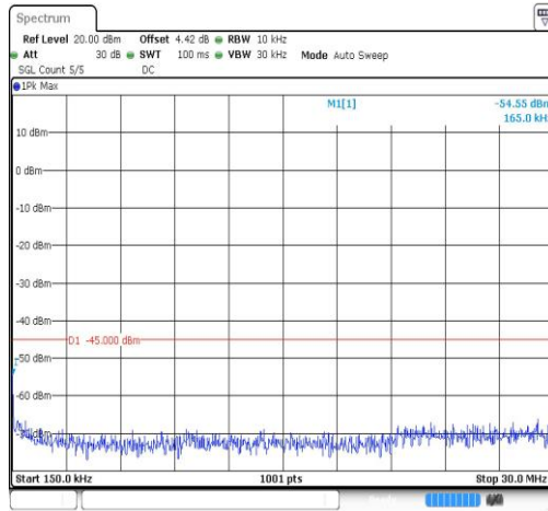
Band38-20MHz-QPSK-38000-1RB#0-Range2:0.15~30MHz
