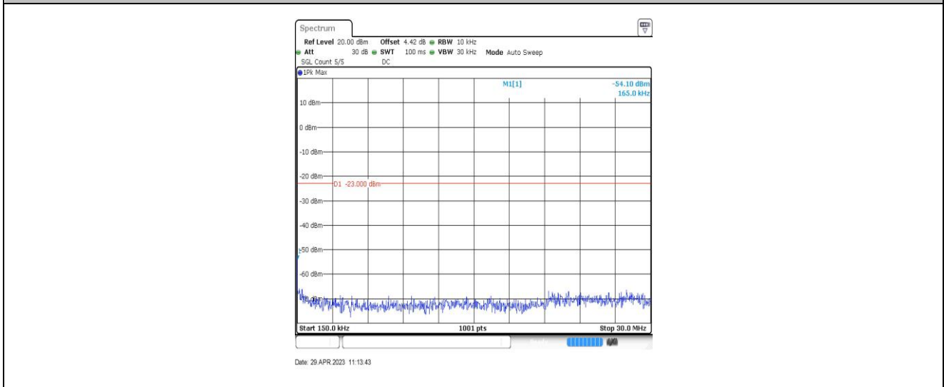
Band26-10MHz-QPSK-26740-1RB#0-Range2:0.15~30MHz
