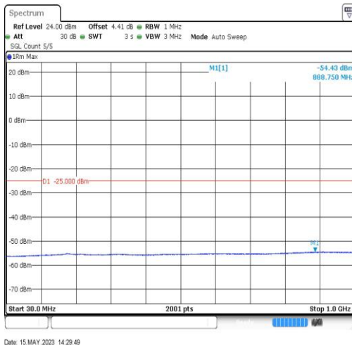
41-41-20MHz-20MHz-QPSK-QPSK-41292-41490-1RB#0-0RB#0-30~1000MHz
