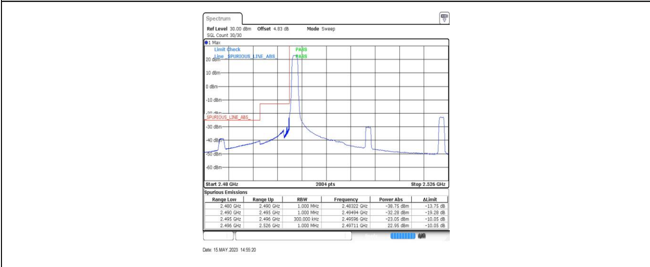
41-41-10MHz-20MHz-QPSK-QPSK-39705-39849-1RB#0-0RB#0
