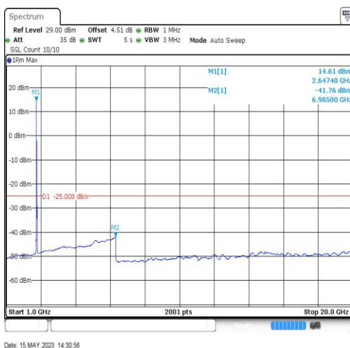
41-41-20MHz-20MHz-QPSK-QPSK-41292-41490-1RB#0-0RB#0-1000~20000MHz
