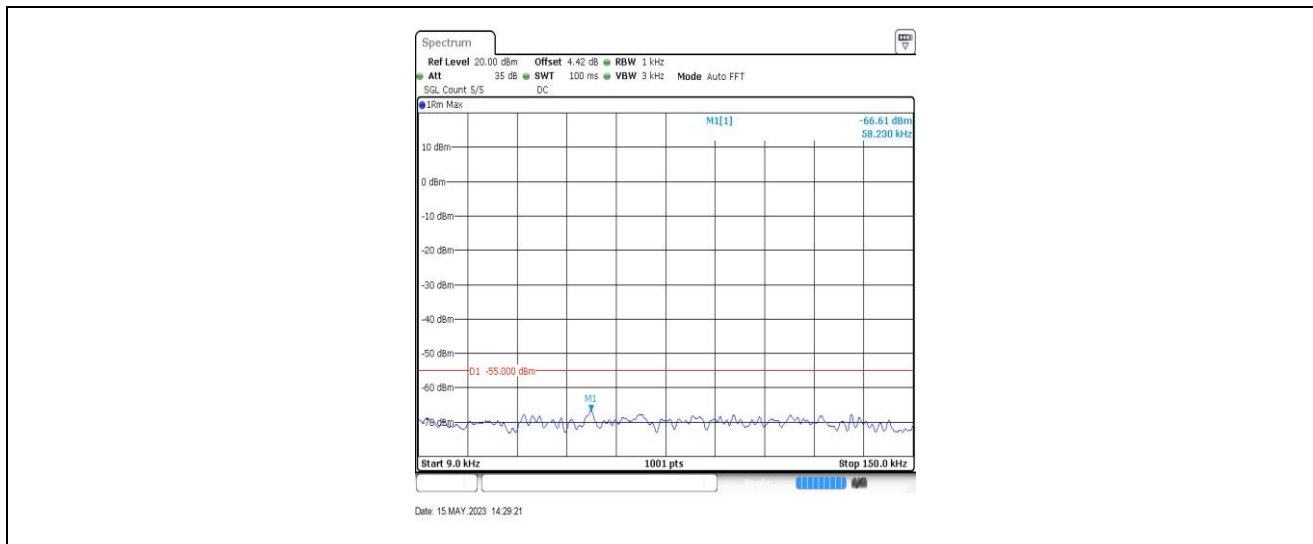
41-41-20MHz-20MHz-QPSK-QPSK-41292-41490-1RB#0-0RB#0-0.009~0.15MHz
