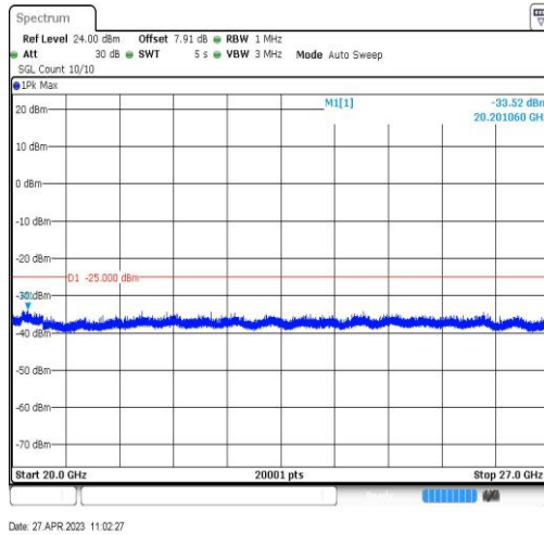
Band7-20MHz-QPSK-21350-1RB#0-Range5:20000~27000MHz
