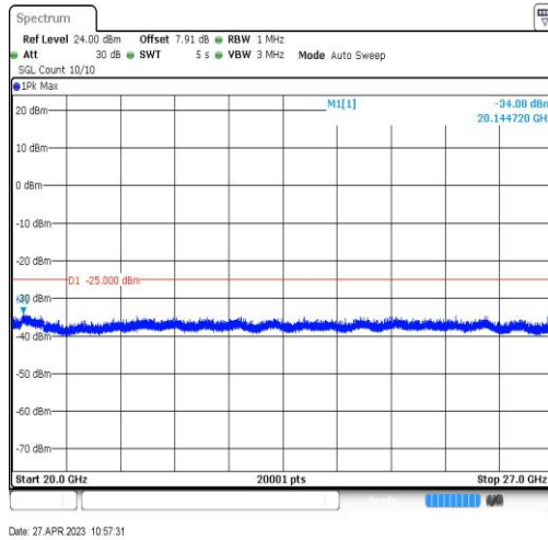
Band7-20MHz-QPSK-20850-1RB#0-Range5:20000~27000MHz
