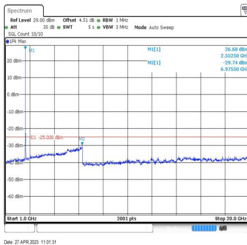
Band7-20MHz-QPSK-21350-1RB#0-Range4:1000~20000MHz
