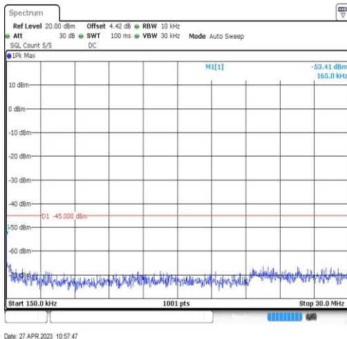
Band7-20MHz-QPSK-21100-1RB#0-Range2:0.15~30MHz
