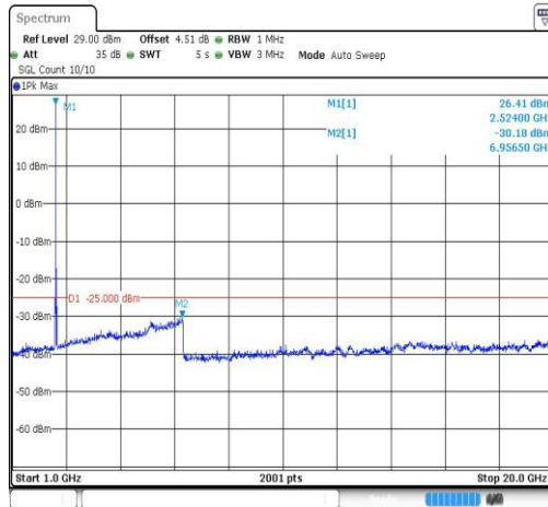
Band7-20MHz-QPSK-21100-1RB#0-Range4:1000~20000MHz
