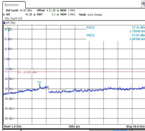
Band4-20MHz-QPSK-20175-1RB#0-Range4: 1000~20000MHz
