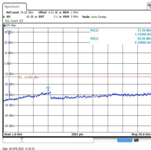
Band4-20MHz-QPSK-20300-1RB#0-Range4:1000~20000MHz
