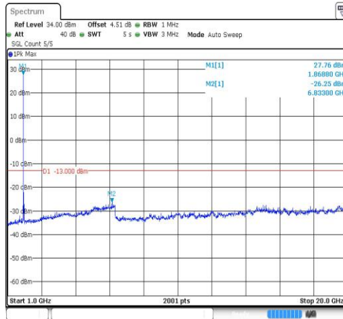
Band2-20MHz-QPSK-18900-1RB#0-Range4:1000~20000MHz
