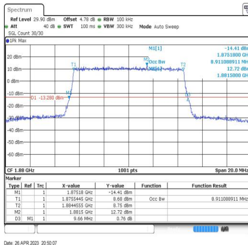
Band2-10MHz-16QAM-18900-50RB#0-8.911
