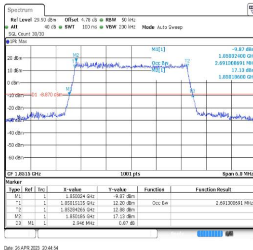
Band2-3MHz-QPSK-18615-15RB#0-2.691
