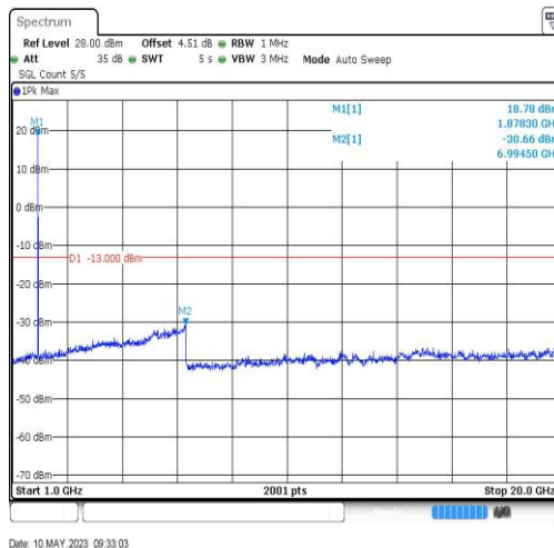
BandII-9400-1000~20000MHz-6994.5
