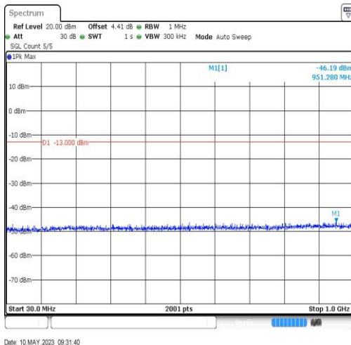
BandII-9262-30~1000MHz-951.28
