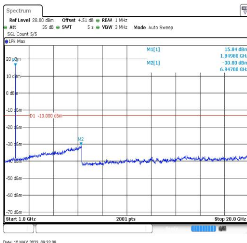
BandII-9262-1000~20000MHz-6947
