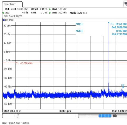
GSM850-251-5-30~1000MHz-959.97
