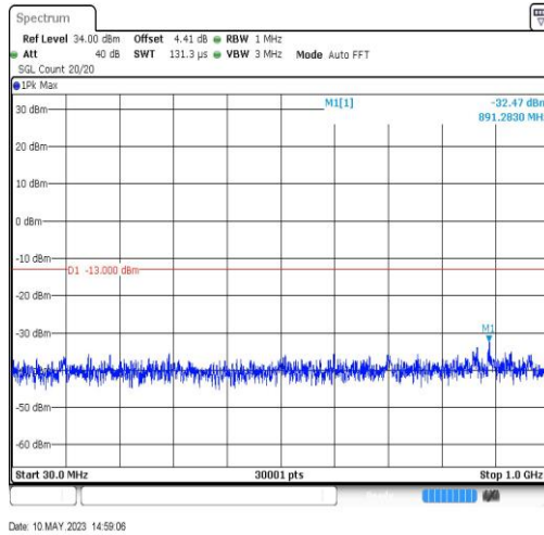
EGPRS1900-810-2-30~1000MHz-891.28
