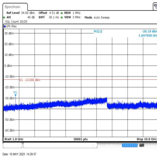
GSM850-251-5-1000~10000MHz-1697.93
