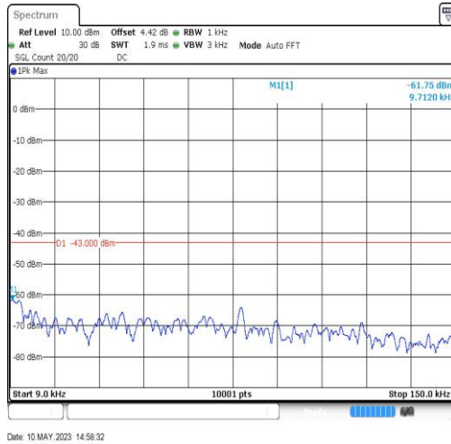
EGPRS1900-661-2-0.009~0.15MHz-0.01
