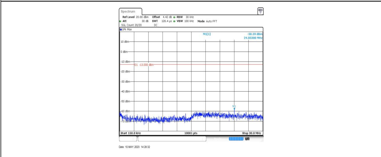
GSM850-128-5-0.15~30MHz-24.05
