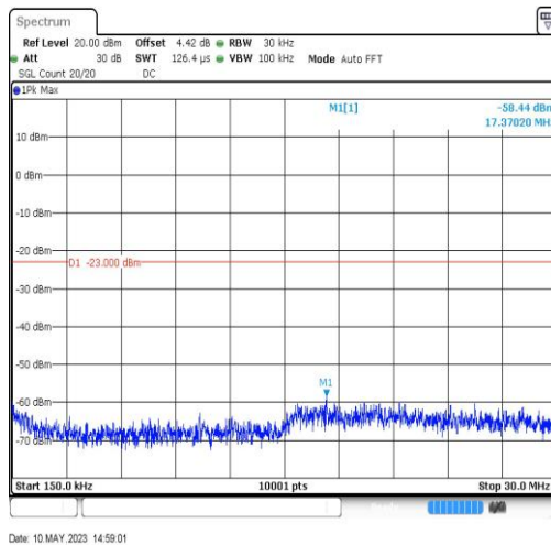
EGPRS1900-810-2-0.15~30MHz-17.37
