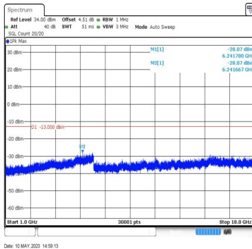
EGPRS1900-810-2-1000~18000MHz-6241.67
