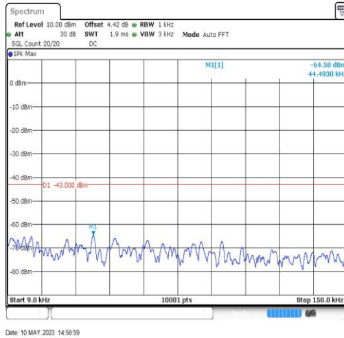
EGPRS1900-810-2-0.009~0.15MHz-0.04
