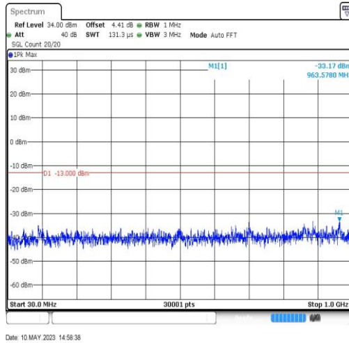
EGPRS1900-661-2-30~1000MHz-963.58
