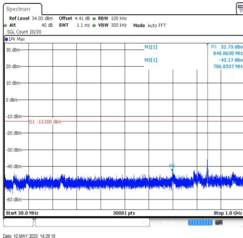
GSM850-190-5-30~1000MHz-706.83
