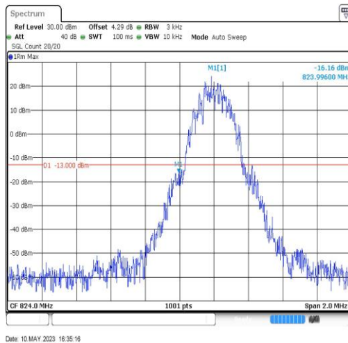
GSM850-128-5-824.00
