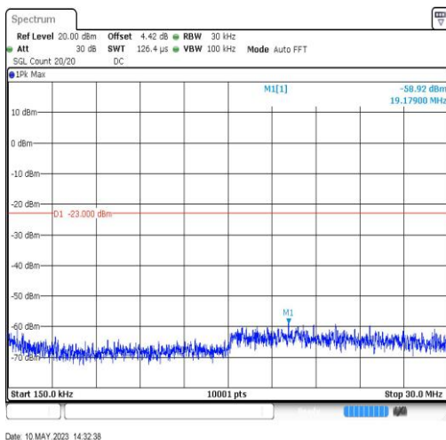
GSM1900-810-0-0.15~30MHz-19.18
