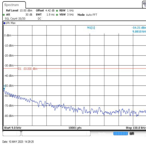
GSM850-251-5-0.009~0.15MHz-0.01
