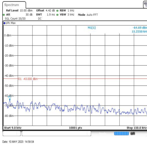
EGPRS1900-512-2-0.009~0.15MHz-0.02
