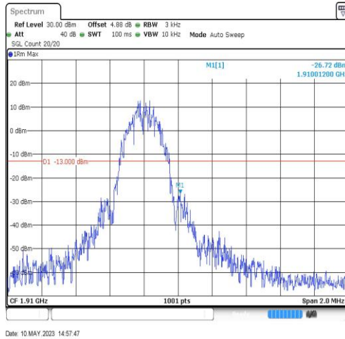
EGPRS1900-810-2-1910.01
