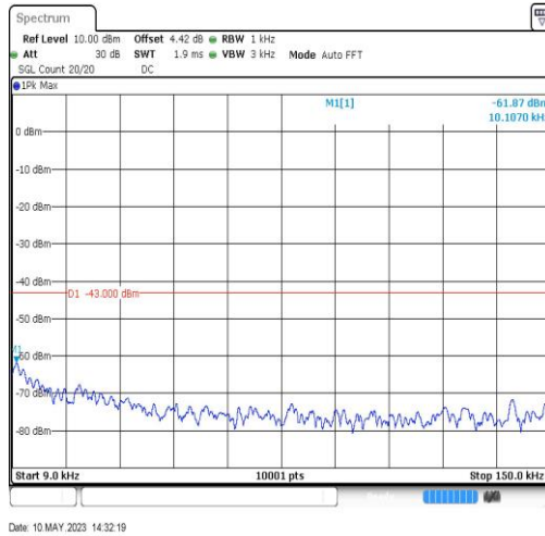
GSM1900-661-0-0.009~0.15MHz-0.01
