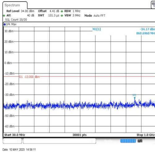
EGPRS1900-512-2-30~1000MHz-860.7
