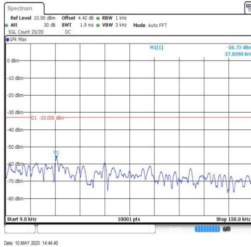
EGPRS850-251-8-0.009~0.15MHz-0.04
