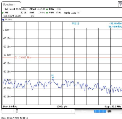
EGPRS850-190-8-0.009~0.15MHz-0.07
