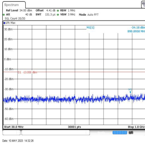
GSM1900-661-0-30~1000MHz-890.9
