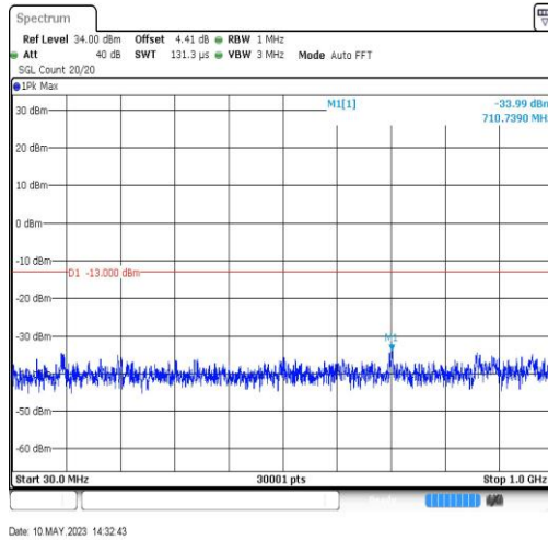
GSM1900-810-0-30~1000MHz-710.74
