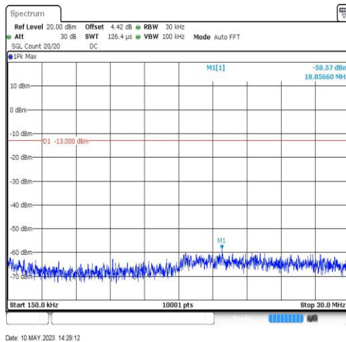
GSM850-190-5-0.15~30MHz-18.86
