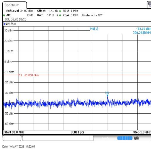
GSM1900-512-0-30~1000MHz-706.25
