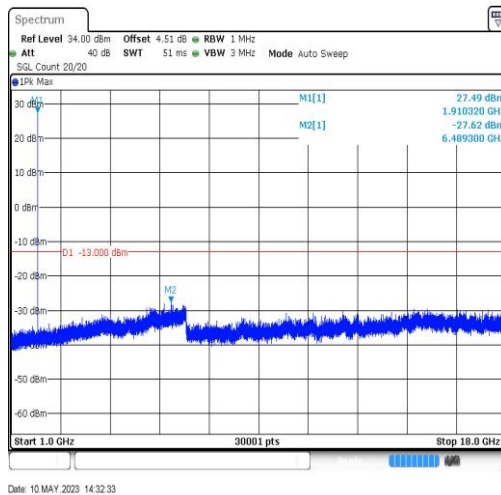
GSM1900-661-0-1000~18000MHz-6489.3
