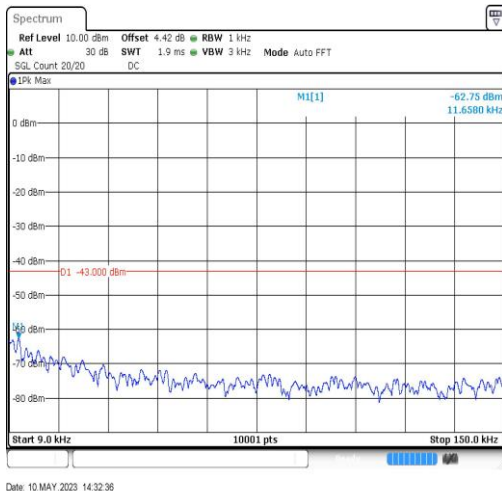
GSM1900-810-0-0.009~0.15MHz-0.01
