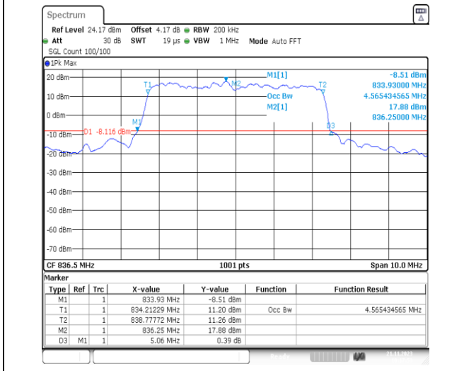
1-N5-PC3-15-5-M-7-CP-16QAM-Outer_Full-25@0-A nt41-4.565-5.060-≤5-PASS
