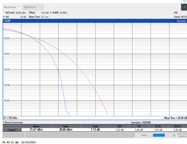
66-66-20MHz-20MHz-QPSK-QPSK-132323-132521-100RB#0-100RB#0
