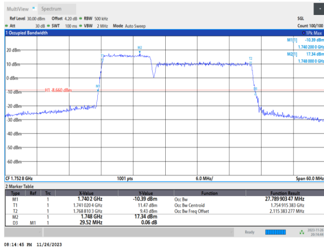
66-66-15MHz-10MHz-QPSK-QPSK-132373-132493-75RB#0-50RB#0
