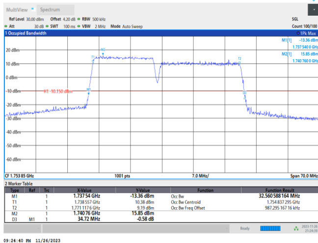
66-66-20MHz-10MHz-QPSK-QPSK-132373-132517-100RB#0-50RB#0
