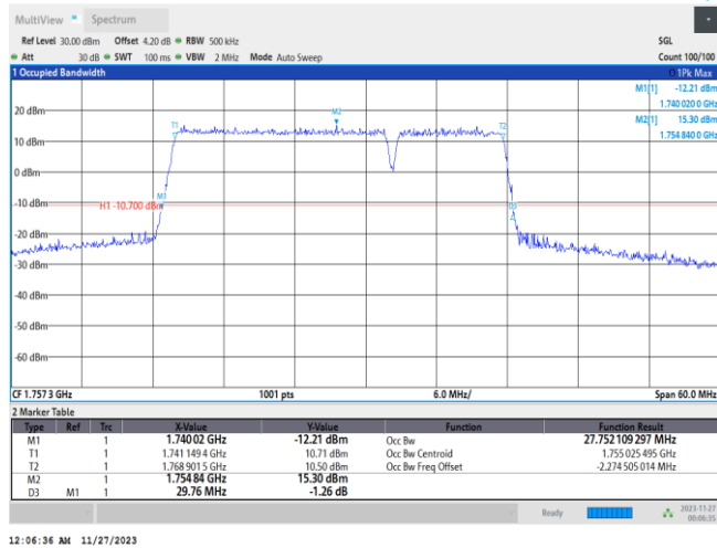
66-66-20MHz-15MHz-QPSK-QPSK-132348-132519-100RB#0-75RB#0
