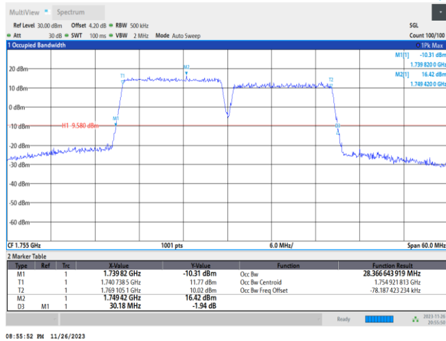
66-66-15MHz-20MHz-QPSK-QPSK-132325-132496-75RB#0-100RB#0
