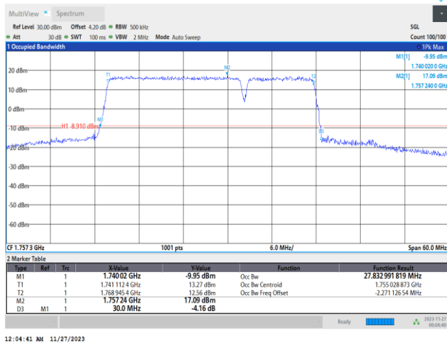
66-66-20MHz-10MHz-16QAM-16QAM-132373-132517-100RB#0-50RB#0
