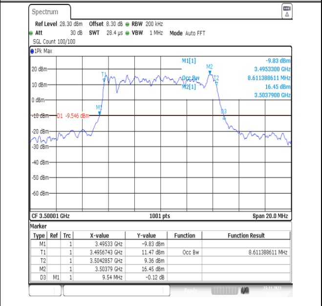
NTNV_N78-3450-3550_PC2_30_10_M_TID8_Ant13#1
