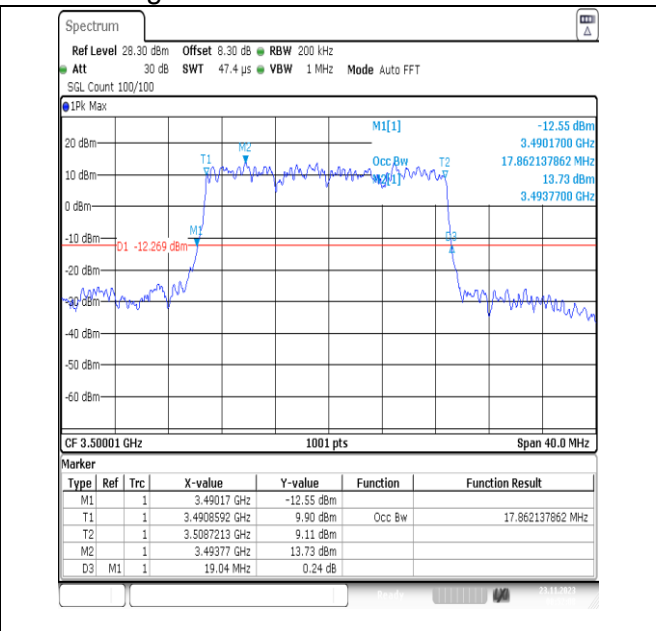
NTNV_N78-3450-3550_PC2_30_20_M_TID4_Ant13#1
