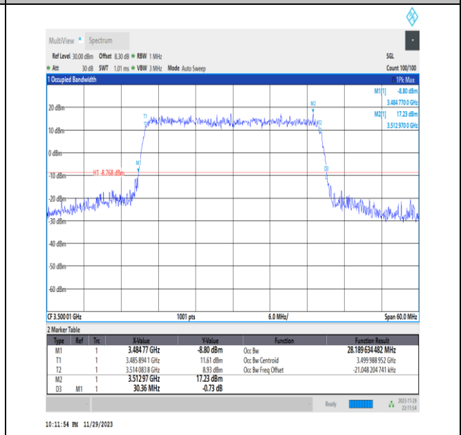
NTNV_N78-3450-3550_PC2_30_30_M_TID9_Ant13#1
