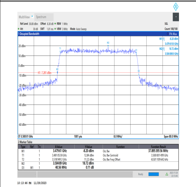
NTNV_N78-3450-3550_PC2_30_40_M_TID8_Ant13#1
