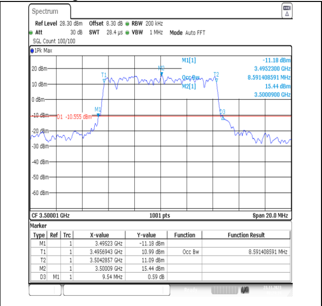
NTNV_N78-3450-3550_PC2_30_10_M_TID6_Ant13#1
