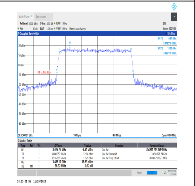
NTNV_N78-3450-3550_PC2_30_40_M_TID4_Ant13#1
