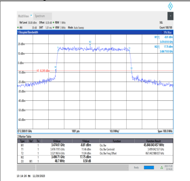
NTNV_N78-3450-3550_PC2_30_50_M_TID1_Ant13#1
