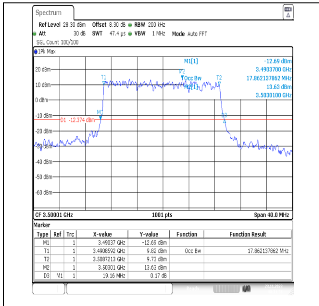
NTNV_N78-3450-3550_PC2_30_20_M_TID3_Ant13#1
