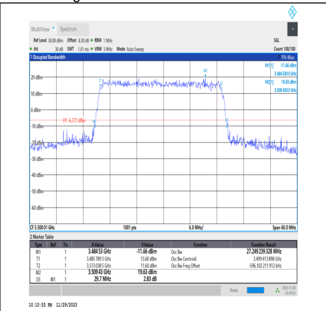
NTNV_N78-3450-3550_PC2_30_30_M_TID3_Ant13#1
