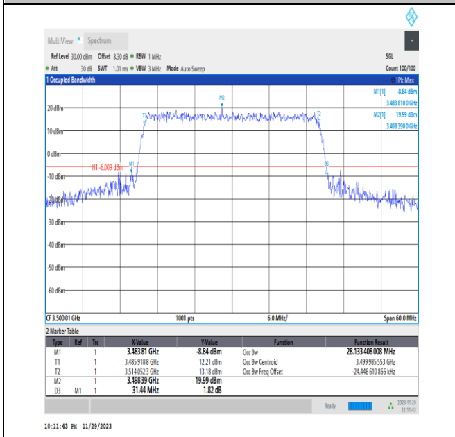
NTNV_N78-3450-3550_PC2_30_30_M_TID8_Ant13#1
