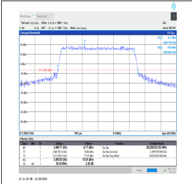
NTNV_N78-3450-3550_PC2_30_30_M_TID6_Ant13#1
