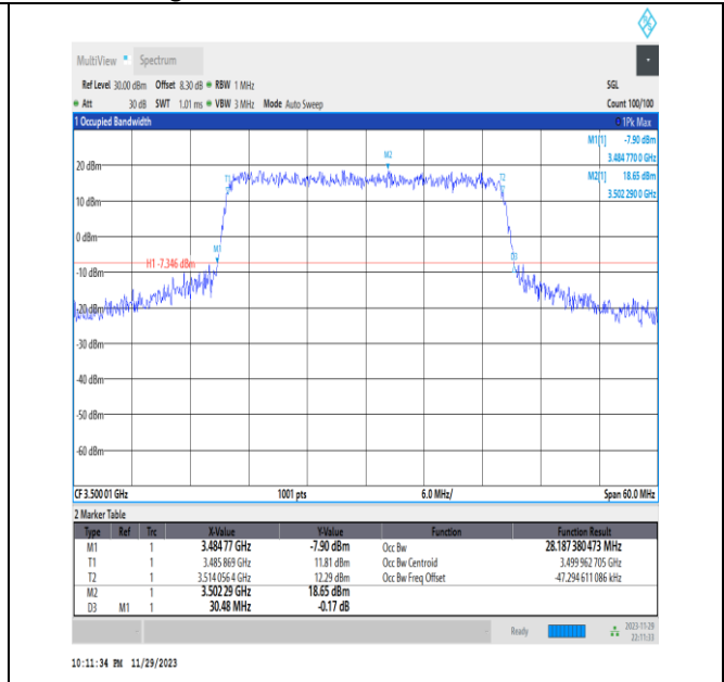
NTNV_N78-3450-3550_PC2_30_30_M_TID7_Ant13#1
