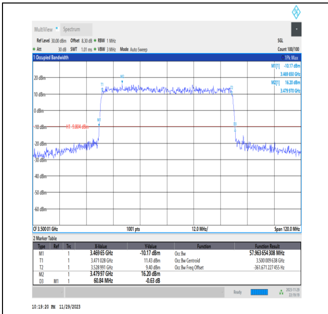
NTNV_N78-3450-3550_PC2_30_60_M_TID3_Ant13#1
