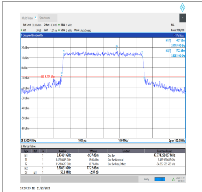
NTNV_N78-3450-3550_PC2_30_50_M_TID8_Ant13#1
