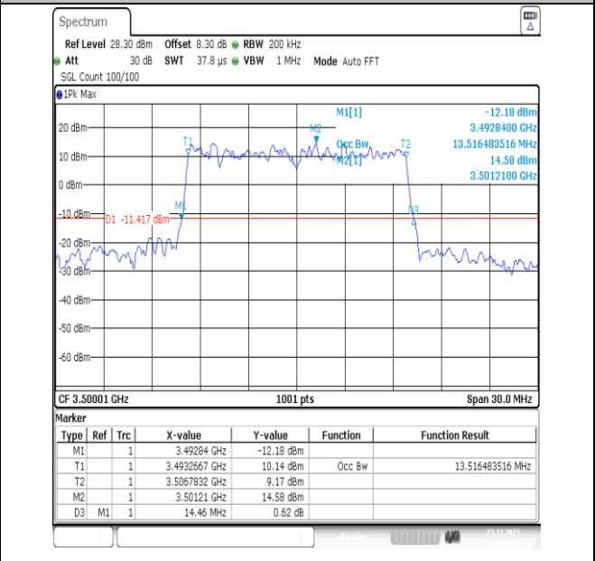
NTNV_N78-3450-3550_PC2_30_15_M_TID7_Ant13#1
