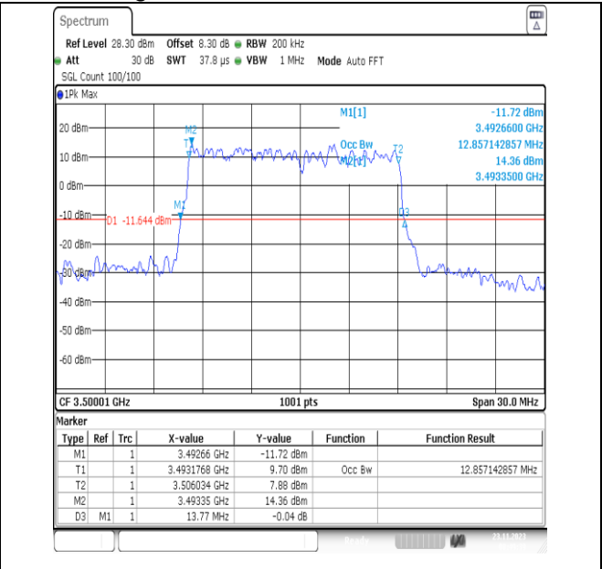
NTNV_N78-3450-3550_PC2_30_15_M_TID5_Ant13#1
