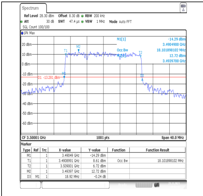
NTNV_N78-3450-3550_PC2_30_20_M_TID7_Ant13#1
