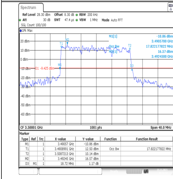
NTNV_N78-3450-3550_PC2_30_20_M_TID1_Ant13#1
