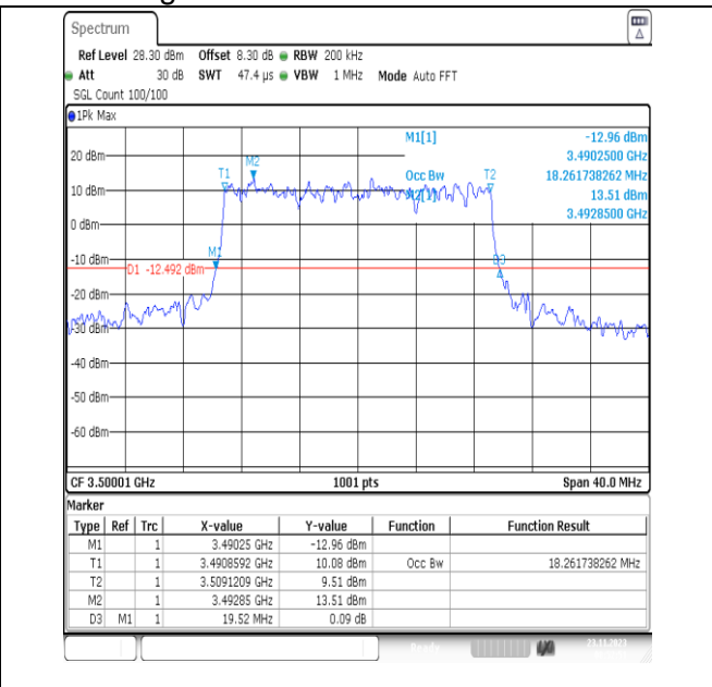
NTNV_N78-3450-3550_PC2_30_20_M_TID8_Ant13#1
