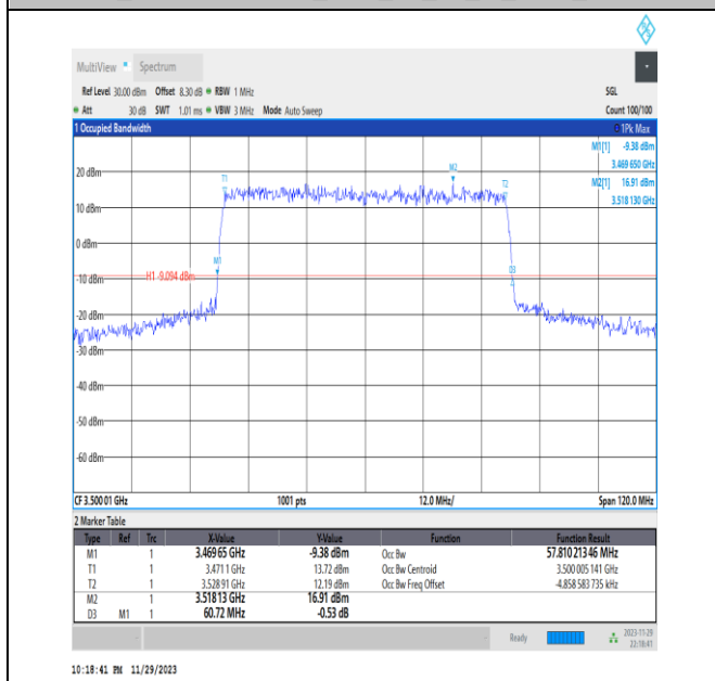
NTNV_N78-3450-3550_PC2_30_60_M_TID1_Ant13#1
