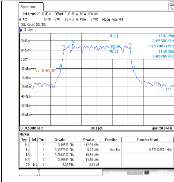
NTNV_N78-3450-3550_PC2_30_10_M_TID5_Ant13#1
