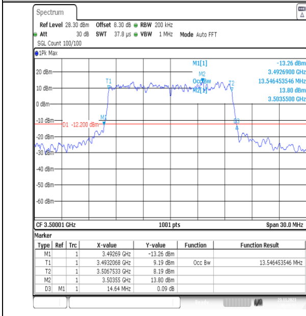
NTNV_N78-3450-3550_PC2_30_15_M_TID6_Ant13#1
