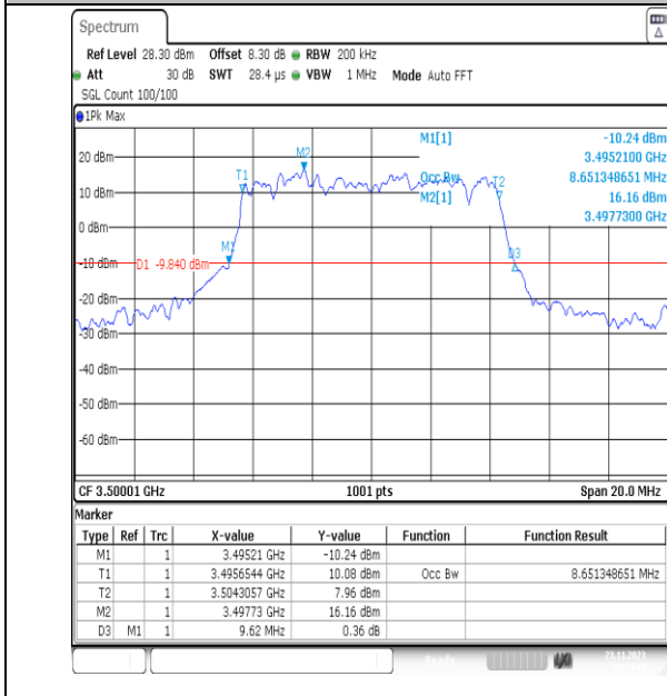
NTNV_N78-3450-3550_PC2_30_10_M_TID7_Ant13#1
