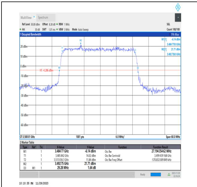
NTNV_N78-3450-3550_PC2_30_30_M_TID2_Ant13#1
