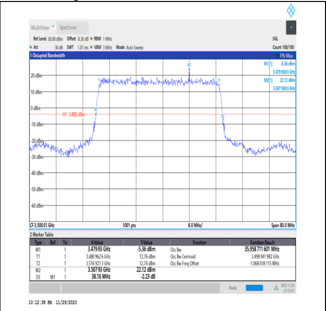
NTNV_N78-3450-3550_PC2_30_40_M_TID2_Ant13#1
