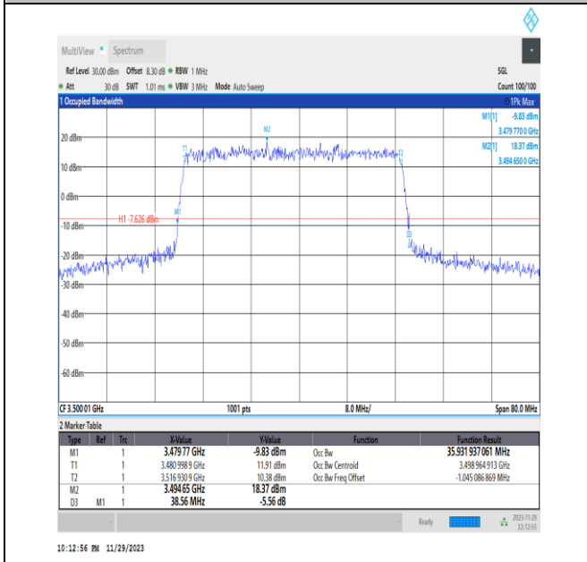
NTNV_N78-3450-3550_PC2_30_40_M_TID3_Ant13#1
