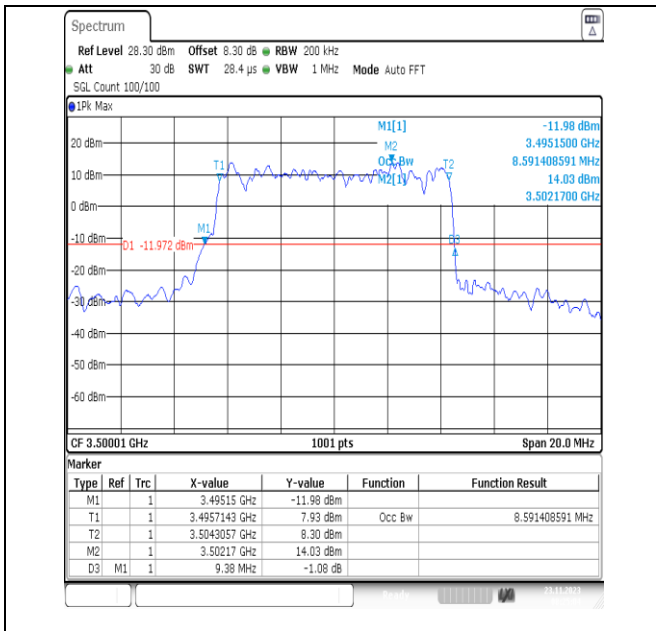
NTNV_N78-3450-3550_PC2_30_10_M_TID9_Ant13#1
