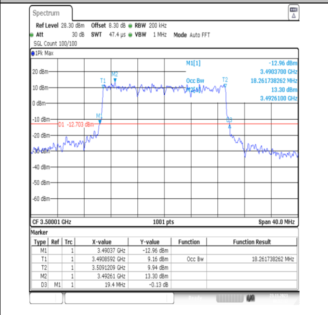
NTNV_N78-3450-3550_PC2_30_20_M_TID6_Ant13#1
