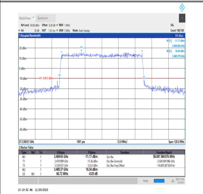
NTNV_N78-3450-3550_PC2_30_60_M_TID6_Ant13#1
