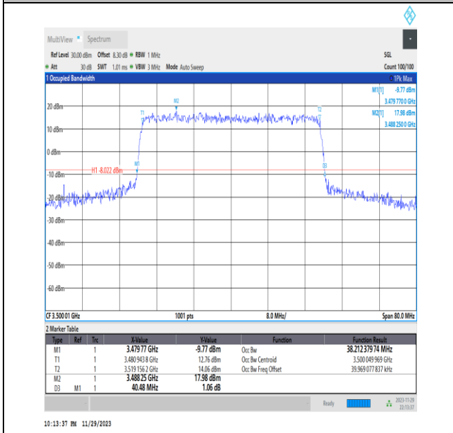
NTNV_N78-3450-3550_PC2_30_40_M_TID7_Ant13#1
