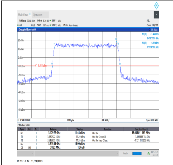
NTNV_N78-3450-3550_PC2_30_40_M_TID5_Ant13#1
