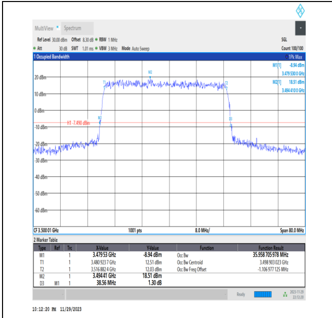
NTNV_N78-3450-3550_PC2_30_40_M_TID1_Ant13#1
