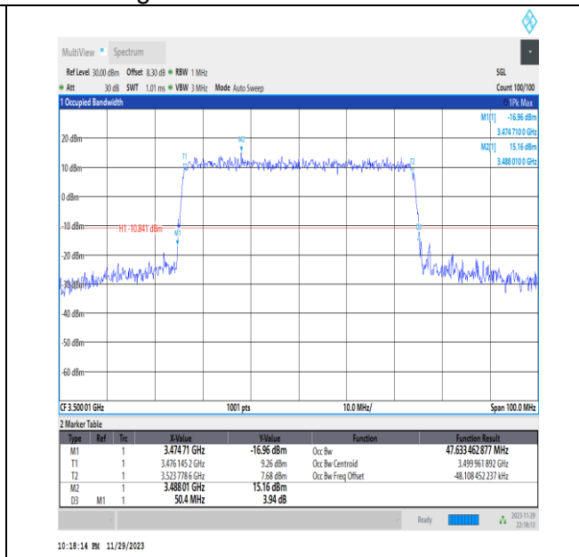
NTNV_N78-3450-3550_PC2_30_50_M_TID9_Ant13#1
