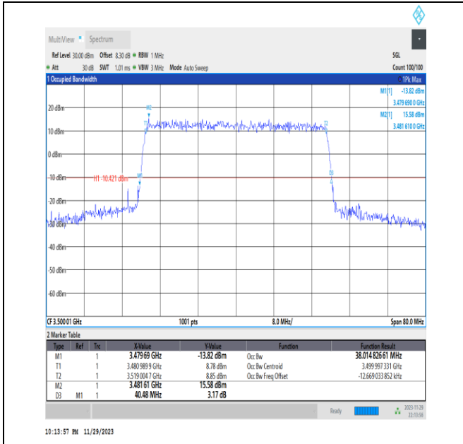
NTNV_N78-3450-3550_PC2_30_40_M_TID9_Ant13#1
