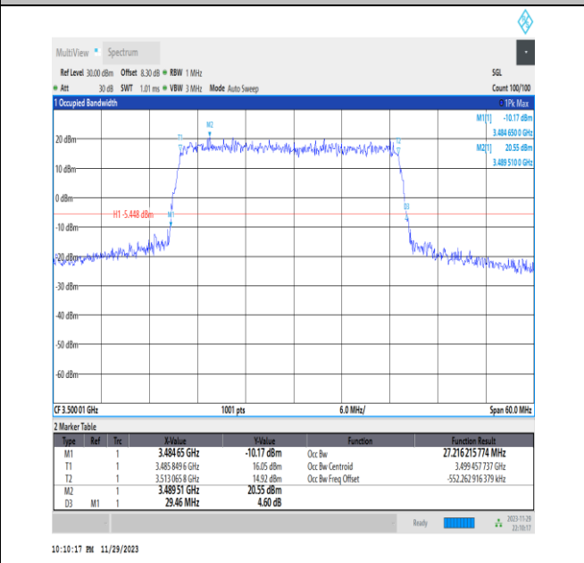
NTNV_N78-3450-3550_PC2_30_30_M_TID1_Ant13#1
