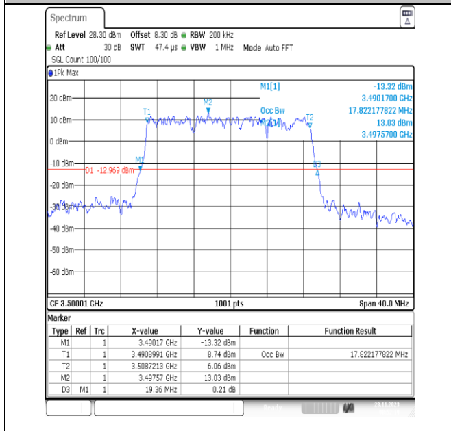
NTNV_N78-3450-3550_PC2_30_20_M_TID5_Ant13#1
