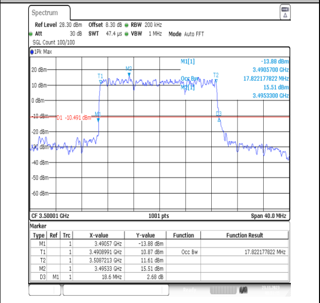
NTNV_N78-3450-3550_PC2_30_20_M_TID2_Ant13#1
