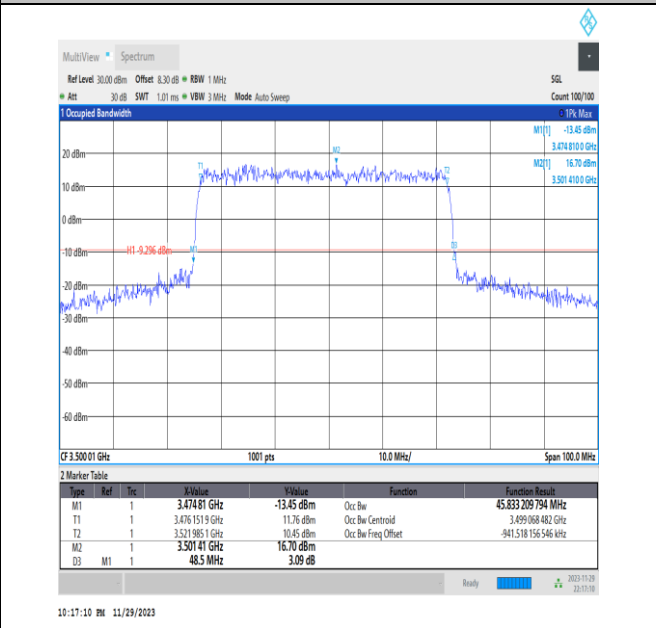
NTNV_N78-3450-3550_PC2_30_50_M_TID3_Ant13#1
