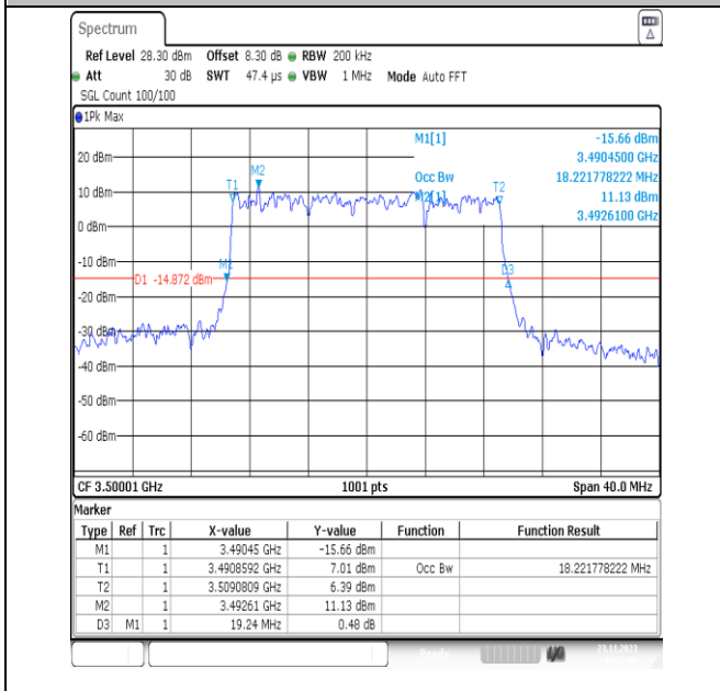
NTNV_N78-3450-3550_PC2_30_20_M_TID9_Ant13#1
