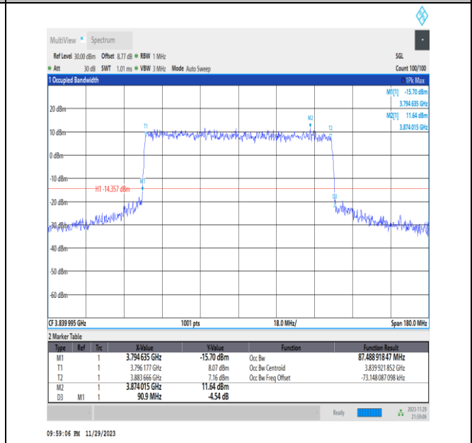
NTNV_N77-3700-3980_PC3_30_90_M_TID7_Ant13#1
