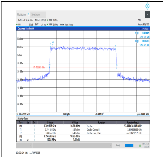
NTVN_N77-3700-3980_PC3_30_100_M_TID7_Ant13#1
