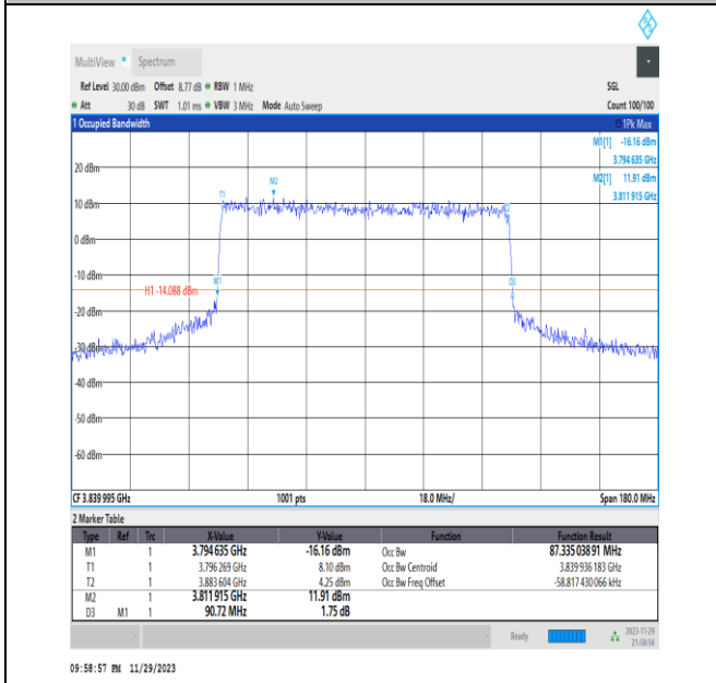
NTNV_N77-3700-3980_PC3_30_90_M_TID6_Ant13#1
