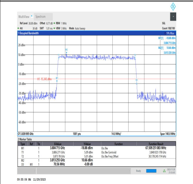
NTNV_N77-3700-3980_PC3_30_70_M_TID9_Ant13#1
