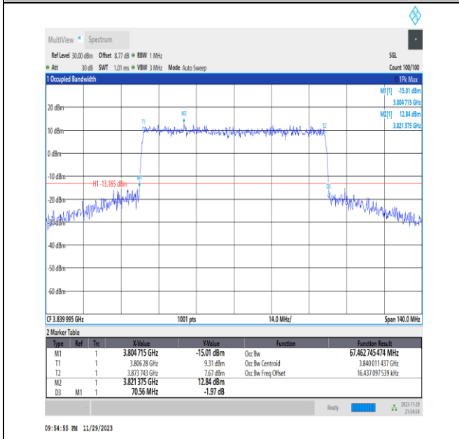
NTNV_N77-3700-3980_PC3_30_70_M_TID8_Ant13#1
