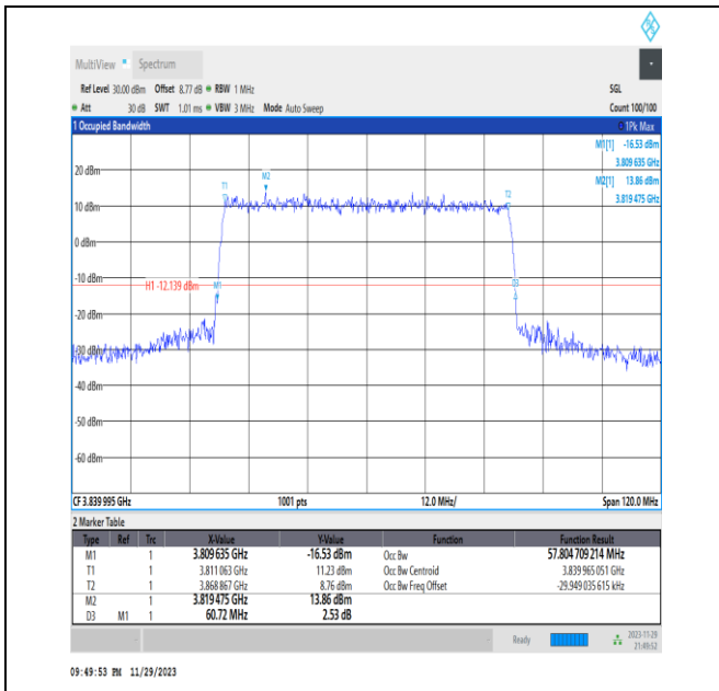
NTNV_N77-3700-3980_PC3_30_60_M_TID3_Ant13#1
