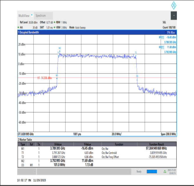
NTVN_N77-3700-3980_PC3_30_100_M_TID6_Ant13#1
