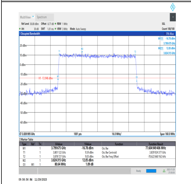
NTNV_N77-3700-3980_PC3_30_80_M_TID7_Ant13#1
