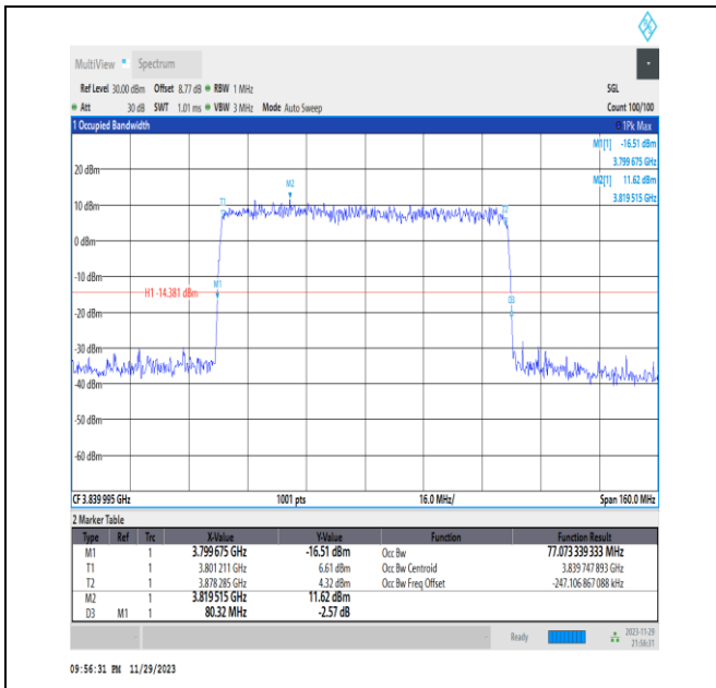
NTNV_N77-3700-3980_PC3_30_80_M_TID5_Ant13#1
