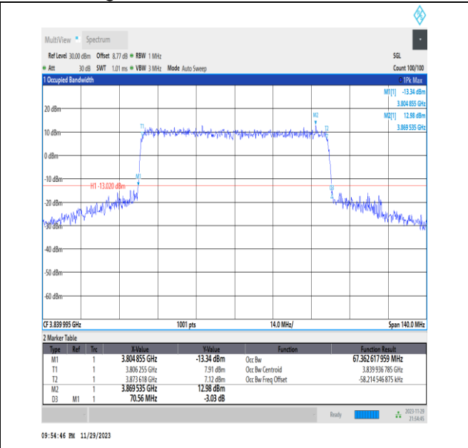
NTNV_N77-3700-3980_PC3_30_70_M_TID7_Ant13#1
