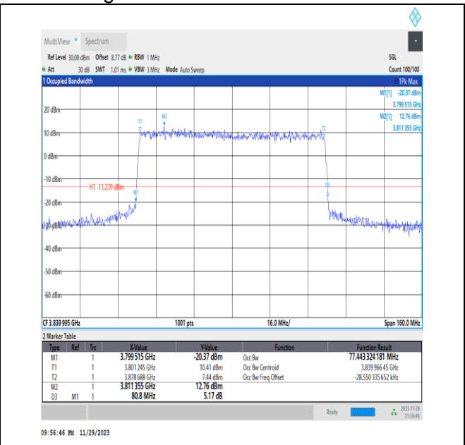
NTNV_N77-3700-3980_PC3_30_80_M_TID6_Ant13#1
