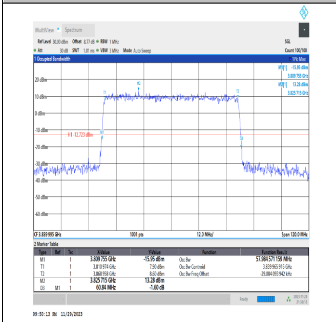
NTNV_N77-3700-3980_PC3_30_60_M_TID5_Ant13#1
