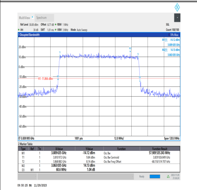
NTNV_N77-3700-3980_PC3_30_60_M_TID6_Ant13#1
