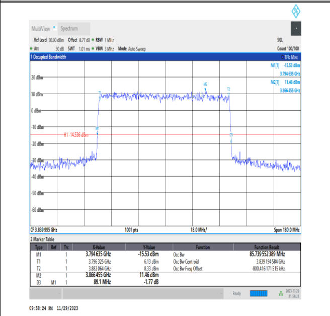
NTNV_N77-3700-3980_PC3_30_90_M_TID3_Ant13#1
