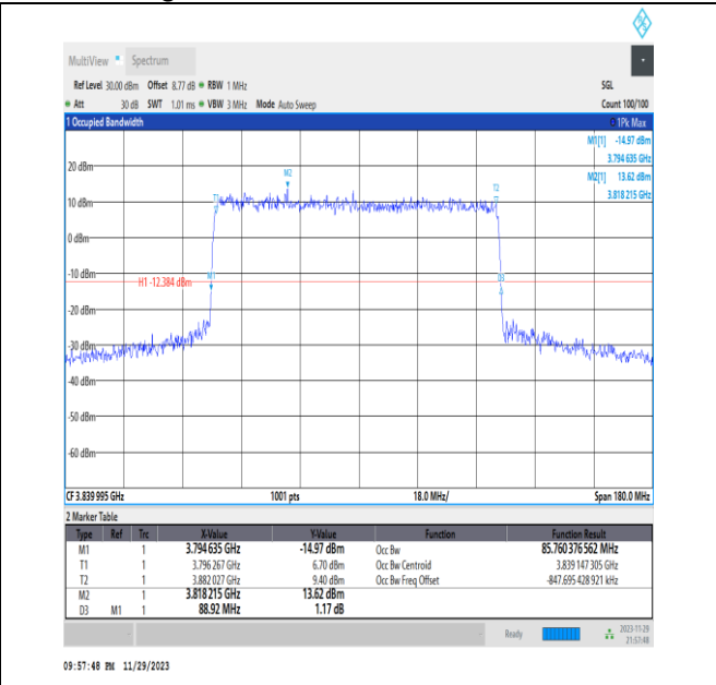
NTNV_N77-3700-3980_PC3_30_90_M_TID1_Ant13#1
