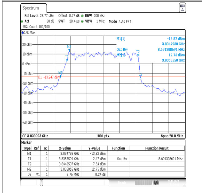
NTNV_N77-3700-3980_PC3_30_10_M_TID7_Ant13#1
