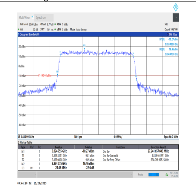
NTNV_N77-3700-3980_PC3_30_30_M_TID7_Ant13#1
