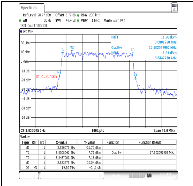
NTNV_N77-3700-3980_PC3_30_20_M_TID3_Ant13#1
