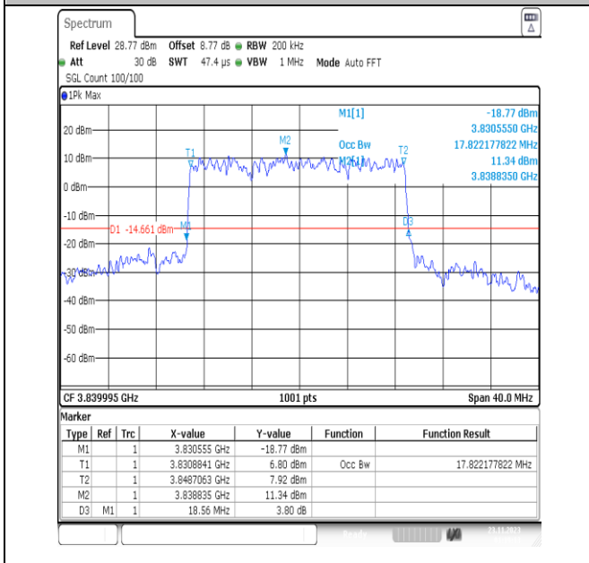
NTNV_N77-3700-3980_PC3_30_20_M_TID1_Ant13#1
