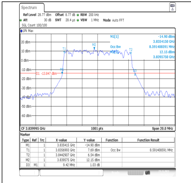
NTNV_N77-3700-3980_PC3_30_10_M_TID5_Ant13#1
