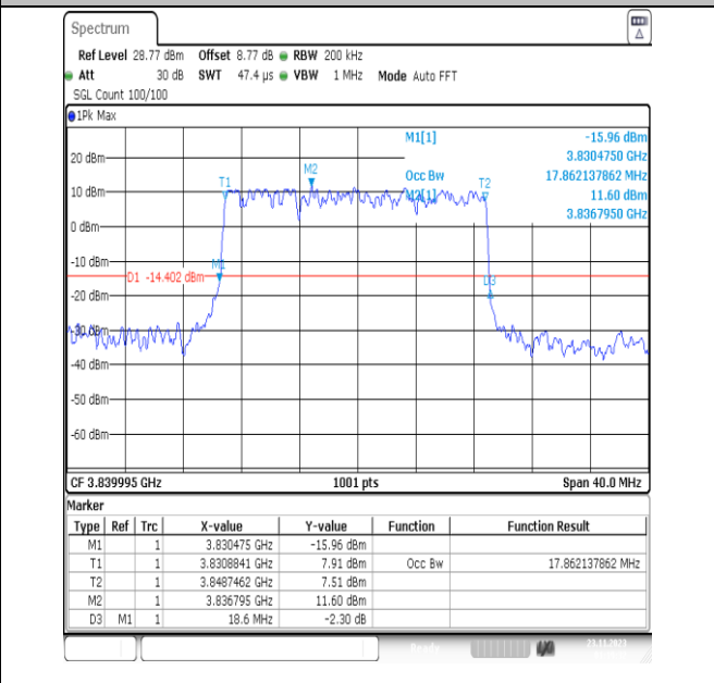
NTNV_N77-3700-3980_PC3_30_20_M_TID2_Ant13#1
