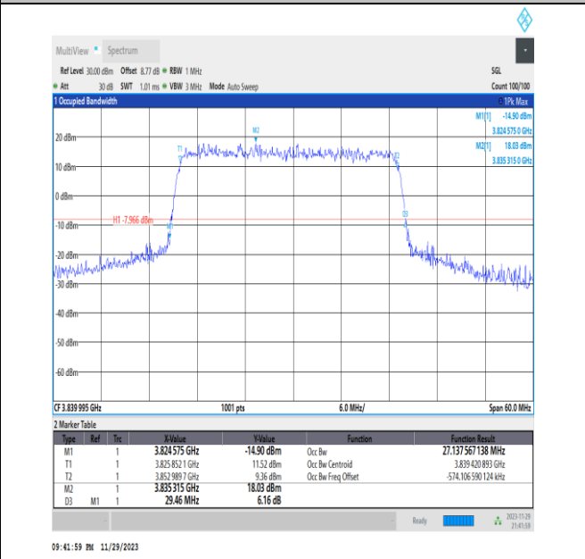
NTNV_N77-3700-3980_PC3_30_30_M_TID1_Ant13#1
