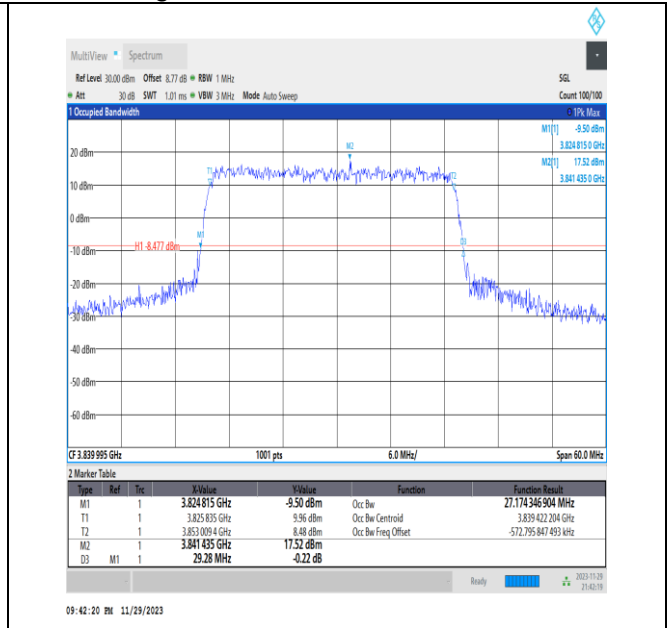
NTNV_N77-3700-3980_PC3_30_30_M_TID3_Ant13#1
