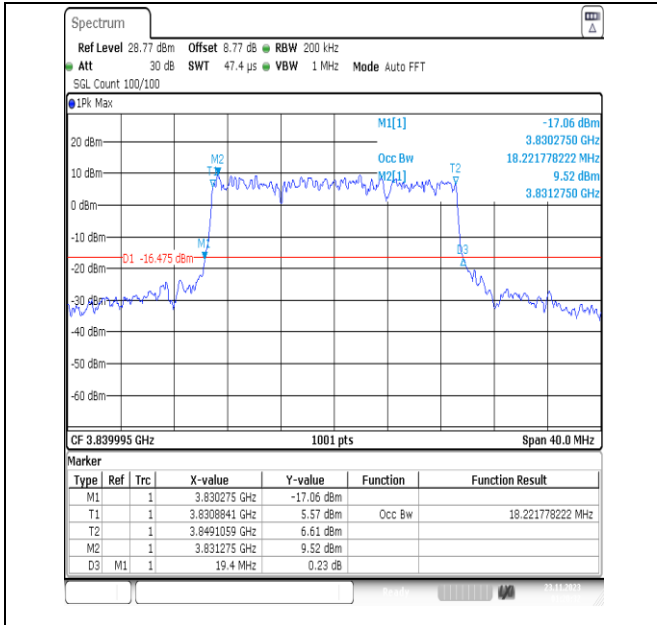
NTNV_N77-3700-3980_PC3_30_20_M_TID7_Ant13#1
