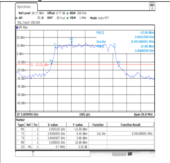
NTNV_N77-3700-3980_PC3_30_10_M_TID6_Ant13#1
