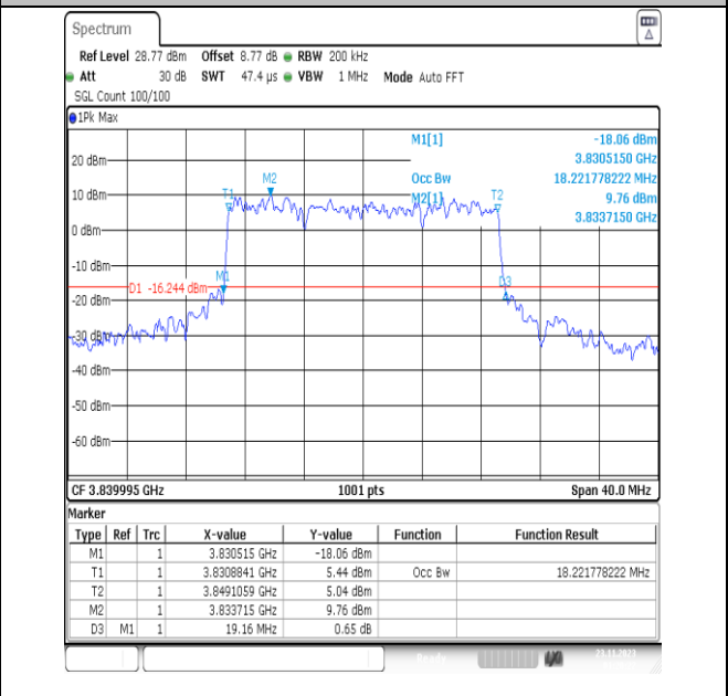
NTNV_N77-3700-3980_PC3_30_20_M_TID6_Ant13#1
