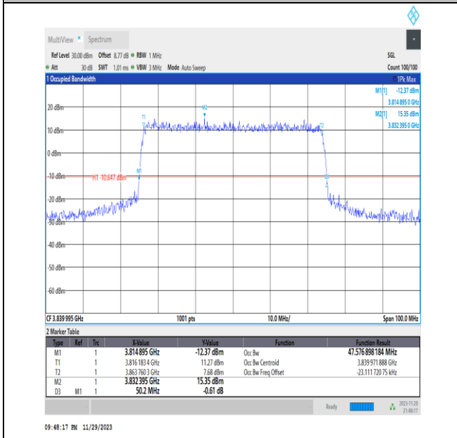
NTNV_N77-3700-3980_PC3_30_50_M_TID6_Ant13#1
