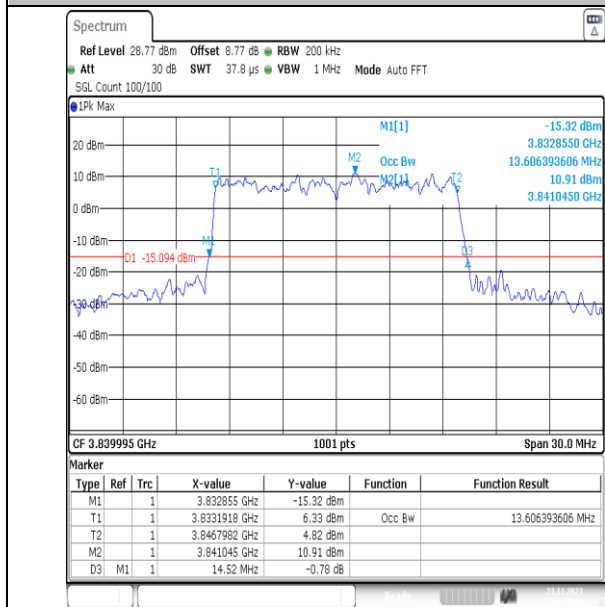
NTNV_N77-3700-3980_PC3_30_15_M_TID6_Ant13#1
