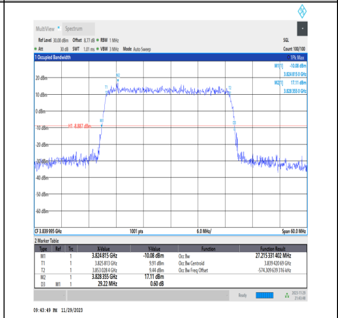
NTNV_N77-3700-3980_PC3_30_30_M_TID5_Ant13#1
