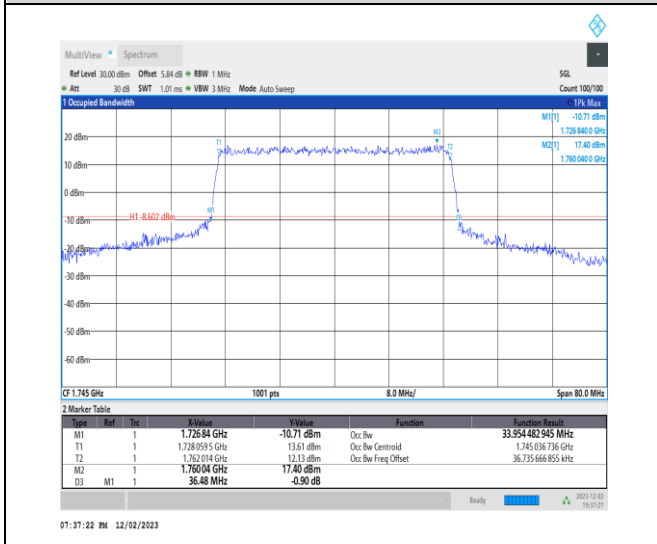
NTNV_N66_PC3_15_35_M_TID9_Ant14#1
