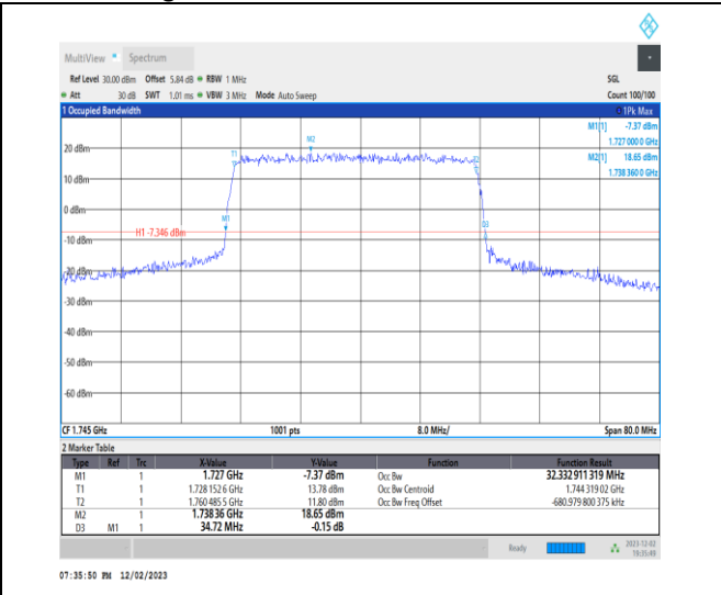
NTVN_N66_PC3_15_35_M_TID4_Ant14#1
