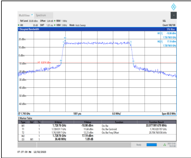
NTNV_N66_PC3_15_35_M_TID7_Ant14#1
