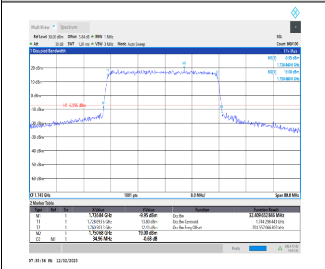
NTVN_N66_PC3_15_35_M_TID5_Ant14#1
