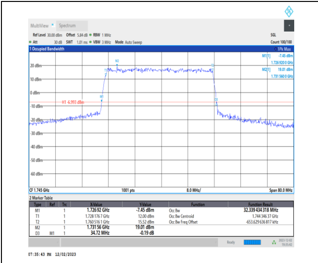
NTVN_N66_PC3_15_35_M_TID3_Ant14#1
