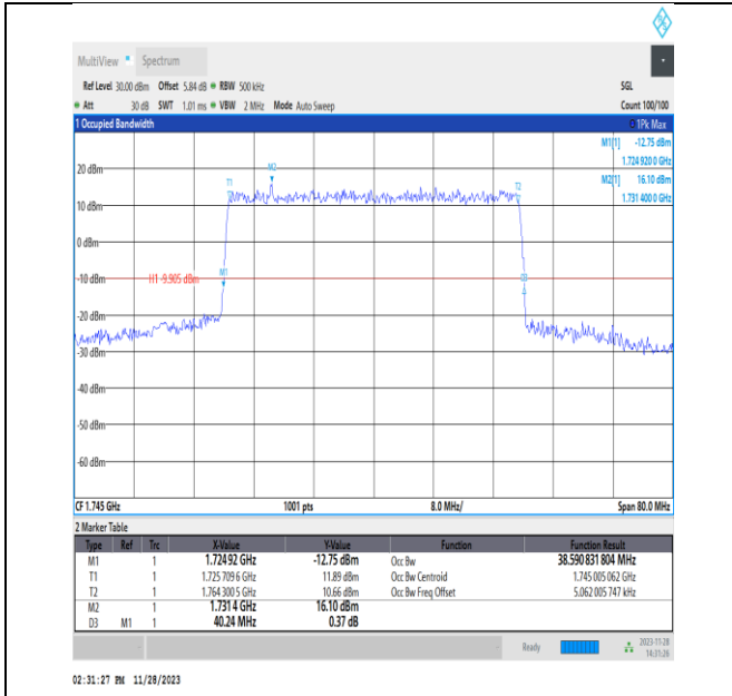
NTNV_N66_PC3_15_40_M_TID1_Ant14#1
