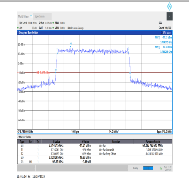
NTNV_N78-3700-3800_PC2_30_70_M_TID1_Ant13#1
