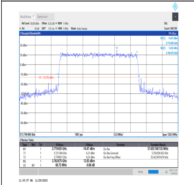
NTNV_N78-3700-3800_PC2_30_60_M_TID9_Ant13#1
