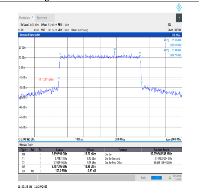
N78-3700-3800_PC2_30_100_M_TID8_Ant13#1
