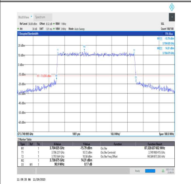
NTNV_N78-3700-3800_PC2_30_90_M_TID7_Ant13#1
