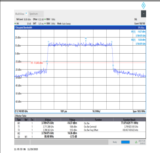
NTNV_N78-3700-3800_PC2_30_80_M_TID4_Ant13#1
