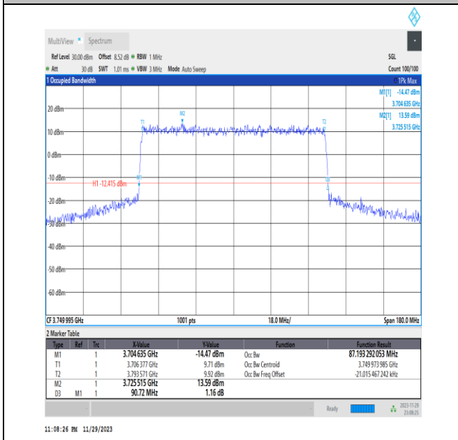
NTNV_N78-3700-3800_PC2_30_90_M_TID6_Ant13#1
