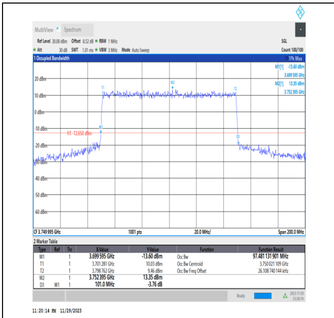
N78-3700-3800_PC2_30_100_M_TID7_Ant13#1
