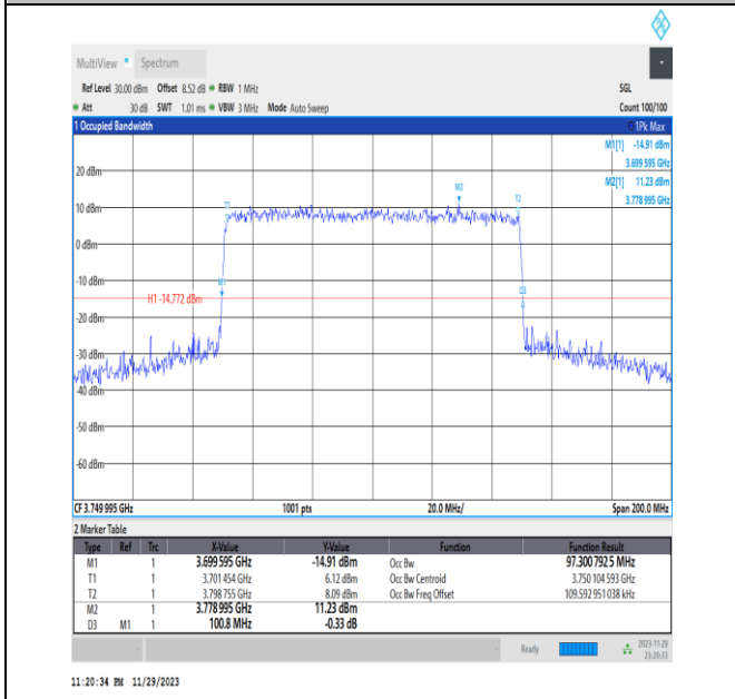
N78-3700-3800_PC2_30_100_M_TID9_Ant13#1
