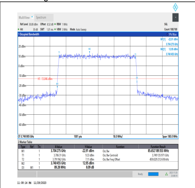
NTNV_N78-3700-3800_PC2_30_90_M_TID5_Ant13#1
