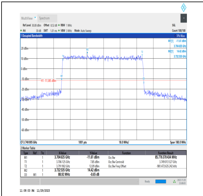
NTNV_N78-3700-3800_PC2_30_90_M_TID4_Ant13#1
