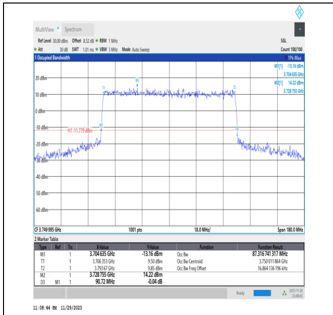
NTNV_N78-3700-3800_PC2_30_90_M_TID8_Ant13#1
