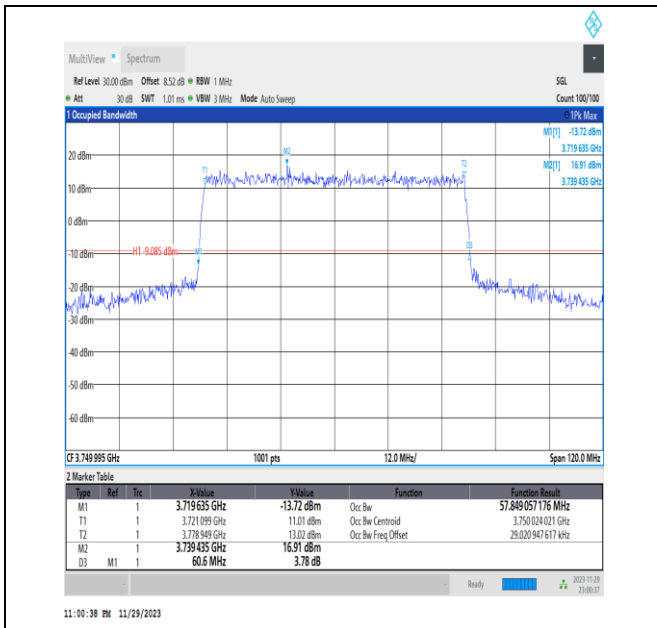
NTNV_N78-3700-3800_PC2_30_60_M_TID7_Ant13#1
