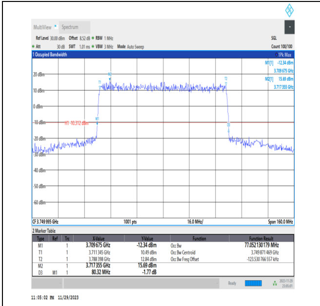
NTNV_N78-3700-3800_PC2_30_80_M_TID1_Ant13#1
