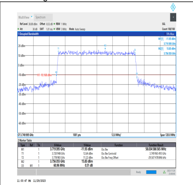
NTNV_N78-3700-3800_PC2_30_60_M_TID8_Ant13#1
