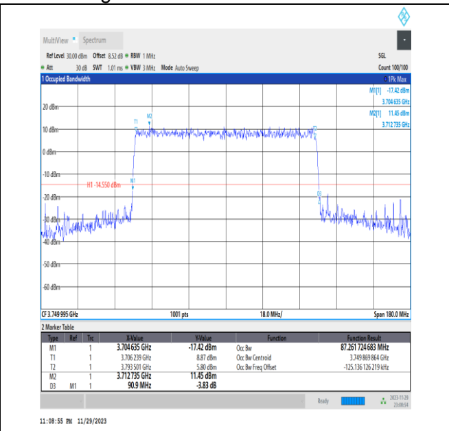
NTNV_N78-3700-3800_PC2_30_90_M_TID9_Ant13#1
