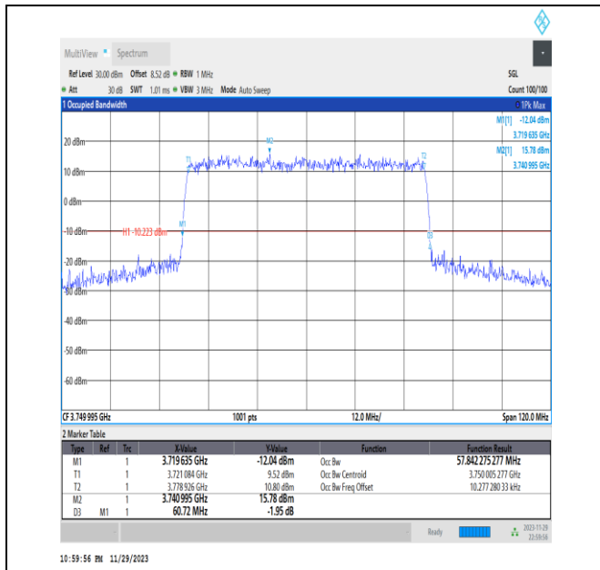
NTNV_N78-3700-3800_PC2_30_60_M_TID3_Ant13#1
