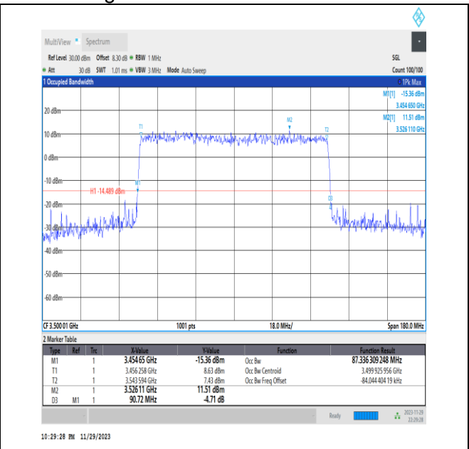
NTNV_N78-3450-3550_PC2_30_90_M_TID9_Ant13#1
