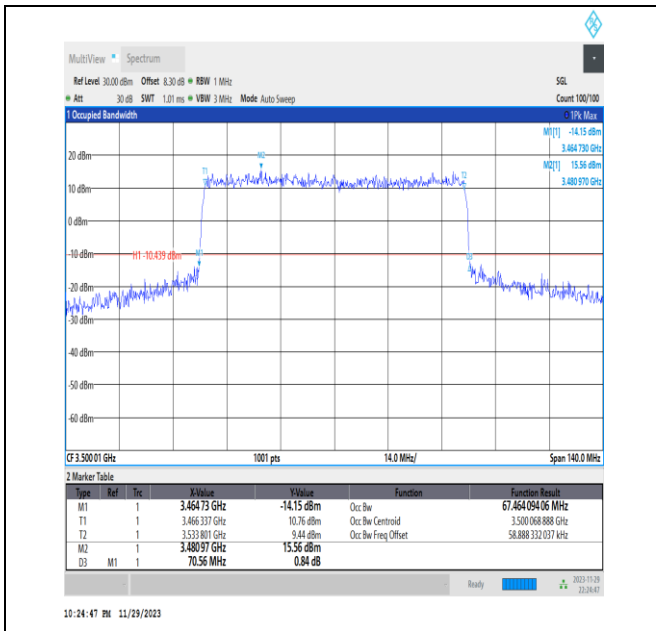
NTNV_N78-3450-3550_PC2_30_70_M_TID6_Ant13#1
