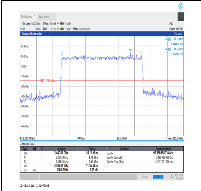
NTVN_N78-3450-3550_PC2_30_100_M_TID9_Ant13#1
