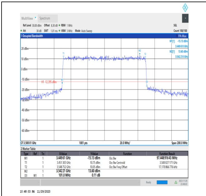
NTVN_N78-3450-3550_PC2_30_100_M_TID7_Ant13#1
