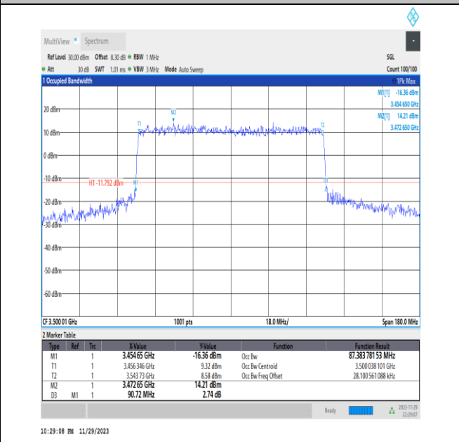
NTNV_N78-3450-3550_PC2_30_90_M_TID7_Ant13#1
