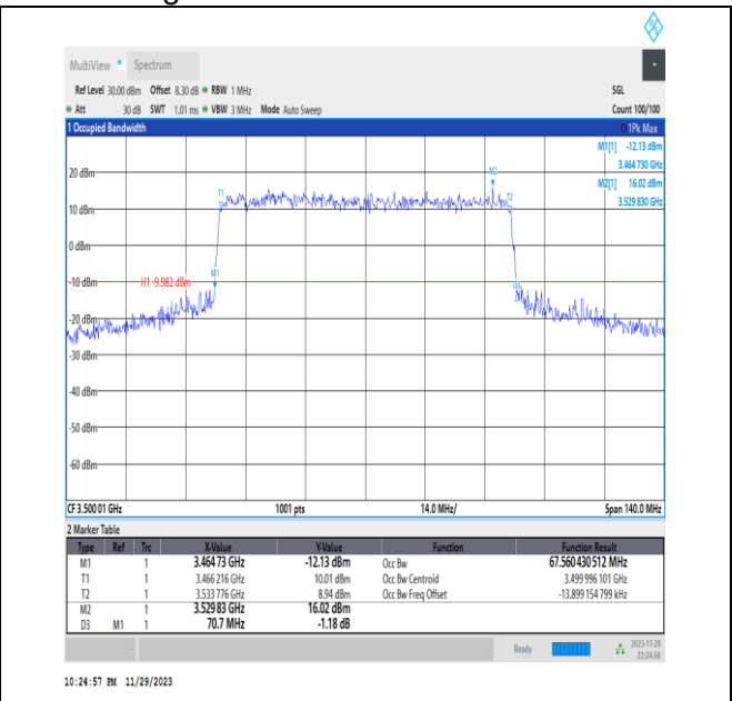
NTNV_N78-3450-3550_PC2_30_70_M_TID7_Ant13#1
