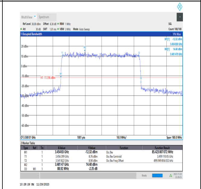
NTNV_N78-3450-3550_PC2_30_90_M_TID3_Ant13#1
