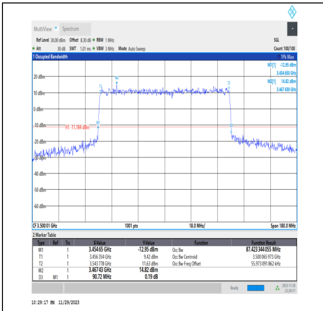
NTNV_N78-3450-3550_PC2_30_90_M_TID8_Ant13#1
