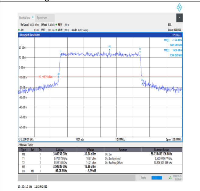
NTNV_N78-3450-3550_PC2_30_60_M_TID8_Ant13#1
