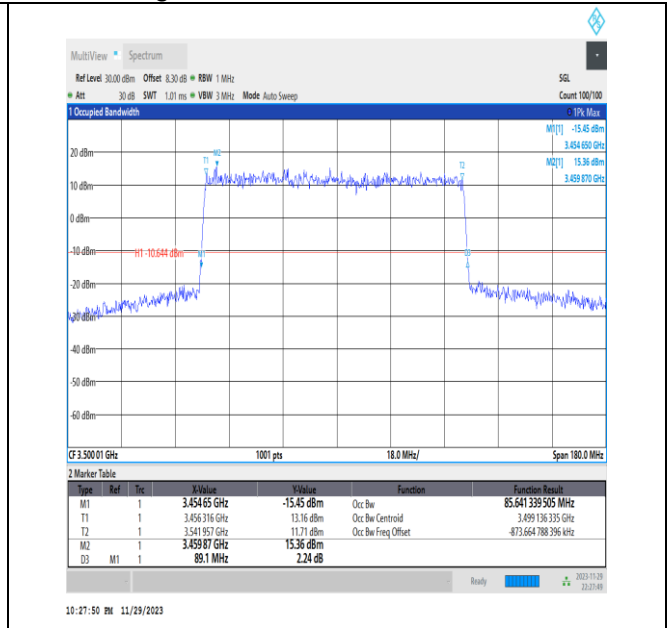
NTNV_N78-3450-3550_PC2_30_90_M_TID1_Ant13#1
