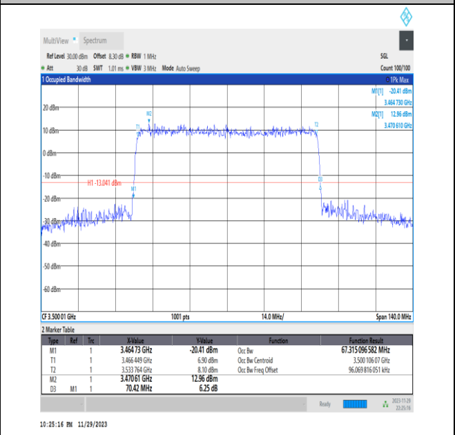
NTNV_N78-3450-3550_PC2_30_70_M_TID9_Ant13#1
