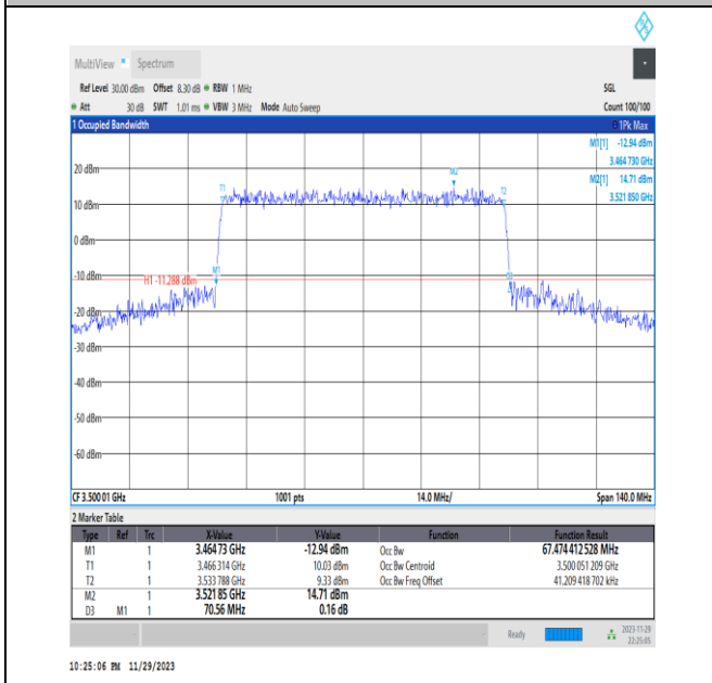
NTNV_N78-3450-3550_PC2_30_70_M_TID8_Ant13#1
