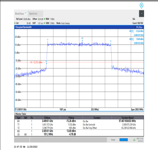
NTVN_N78-3450-3550_PC2_30_100_M_TID6_Ant13#1
