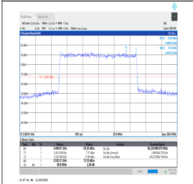
NTVN_N78-3450-3550_PC2_30_100_M_TID5_Ant13#1
