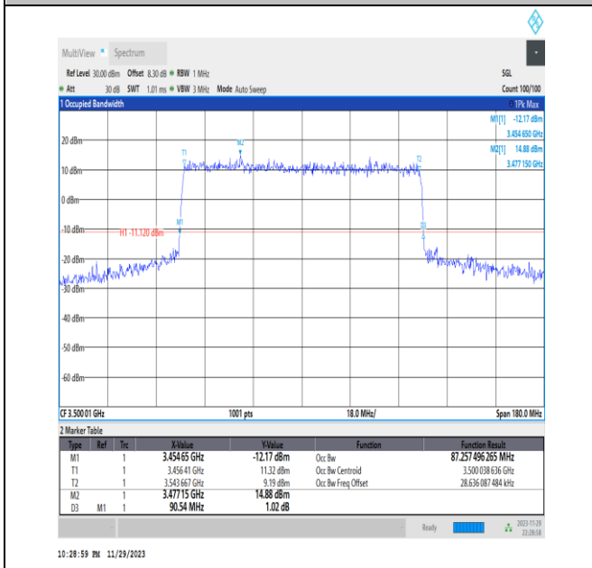
NTNV_N78-3450-3550_PC2_30_90_M_TID6_Ant13#1
