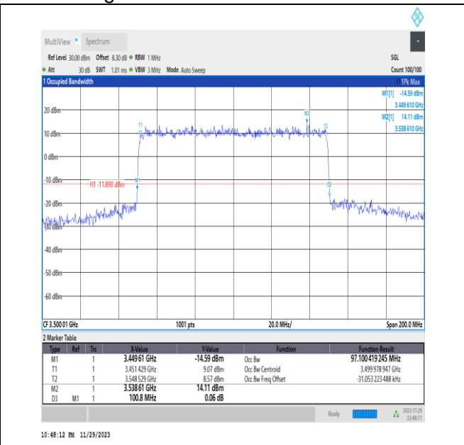
NTVN_N78-3450-3550_PC2_30_100_M_TID8_Ant13#1
