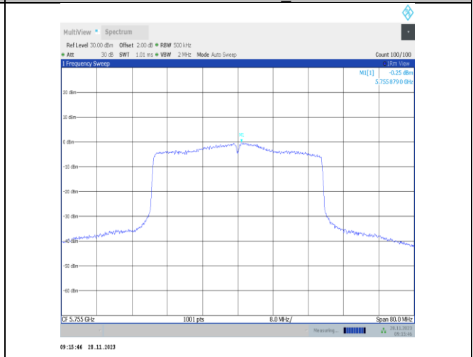
11ax40MIMO-Ant25-5755-PASS
