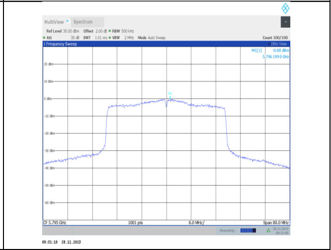
11ax40MIMO-Ant25-5795-PASS
