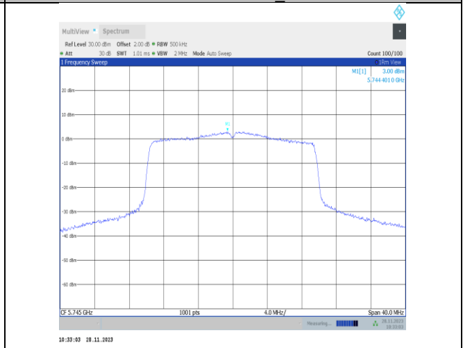
11ax20MIMO-Ant25-5745-PASS
