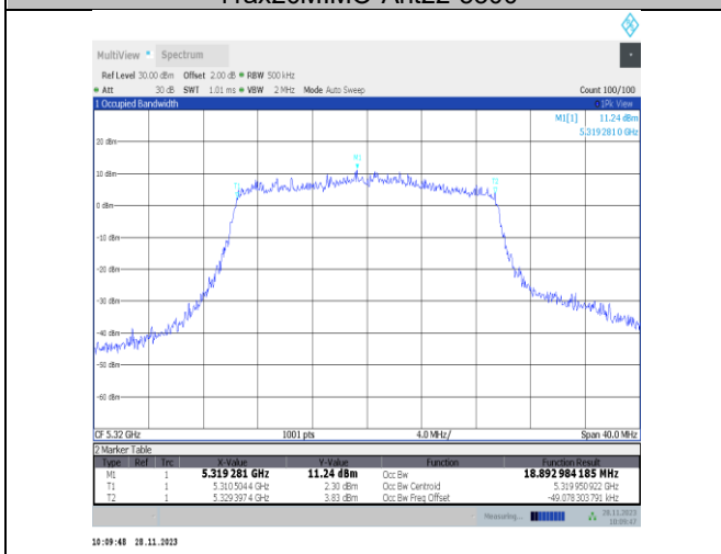
11ax20MIMO-Ant22-5320
