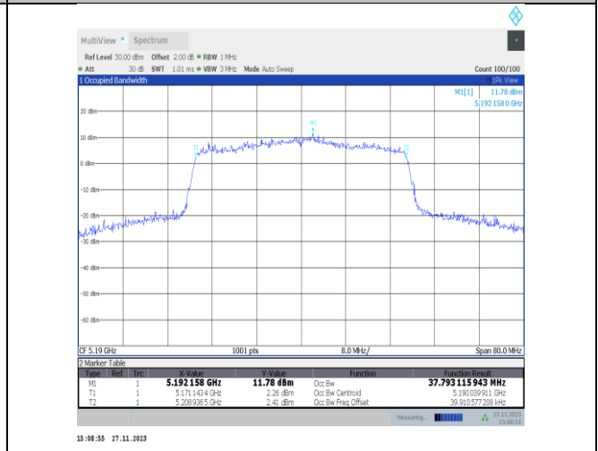
11ax40MIMO-Ant25-5190
