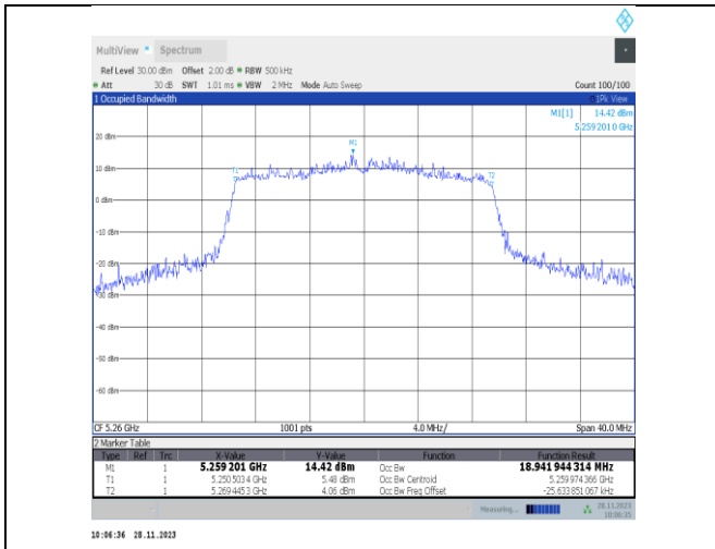
11ax20MIMO-Ant22-5260
