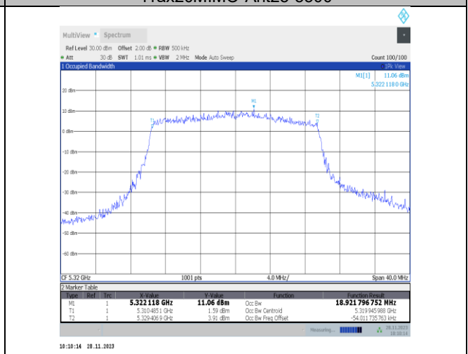
11ax20MIMO-Ant25-5320
