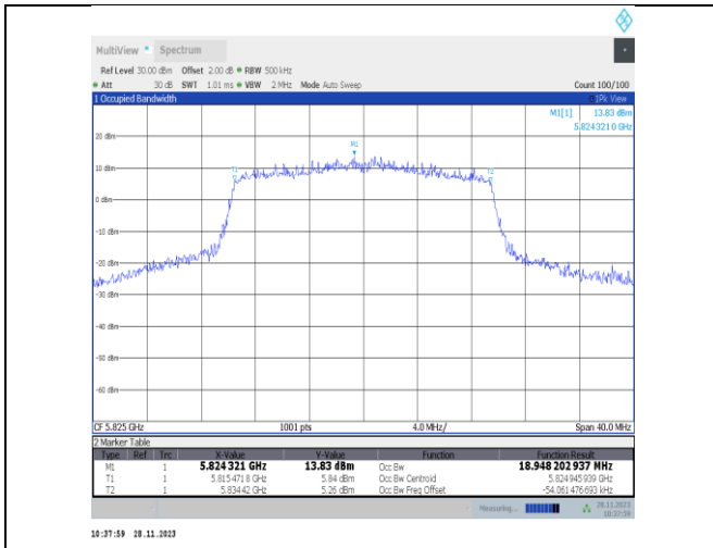
11ax20MIMO-Ant22-5825
