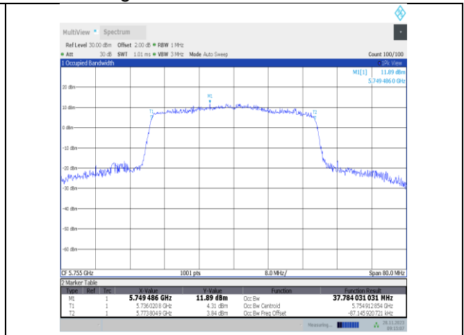
11ax40MIMO-Ant25-5755
