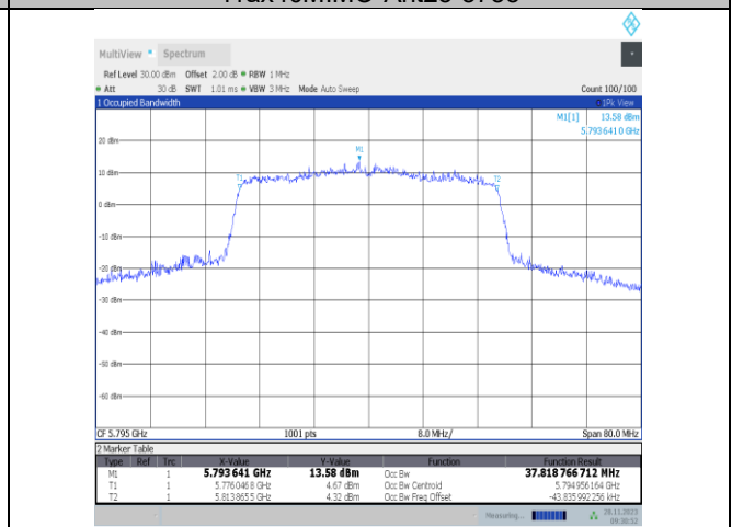
11ax40MIMO-Ant25-5795
