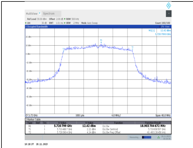
11ax20MIMO-Ant22-5720
