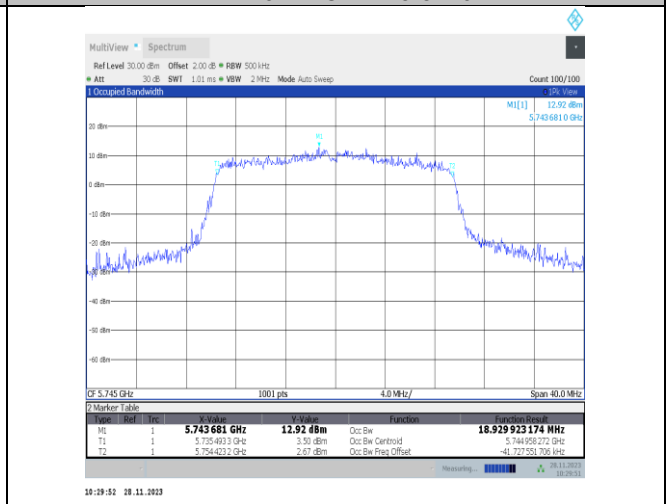
11ax20MIMO-Ant25-5745
