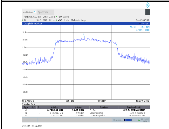
11ax20MIMO-Ant22-5745
