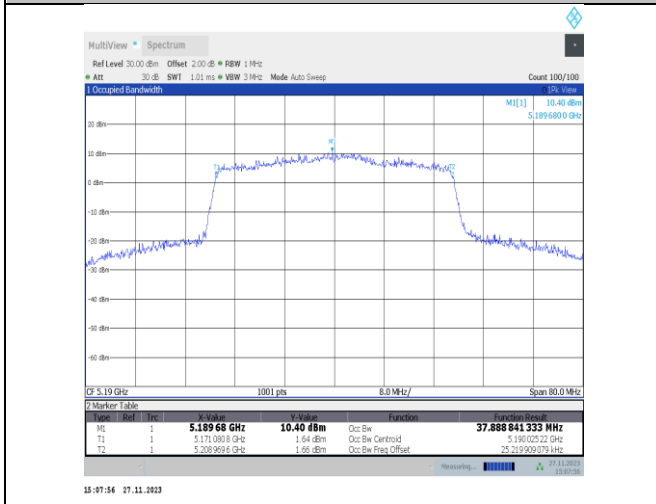
11ax40MIMO-Ant22-5190
