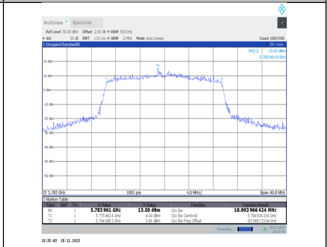
11ax20MIMO-Ant25-5785
