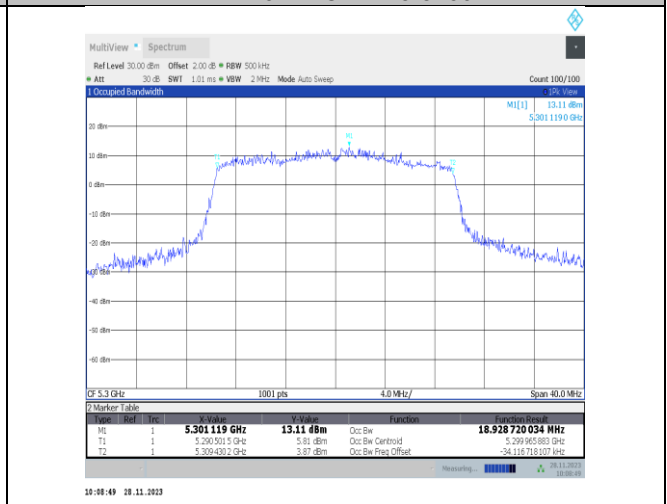
11ax20MIMO-Ant25-5300
