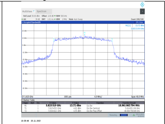
11ax20MIMO-Ant25-5825
