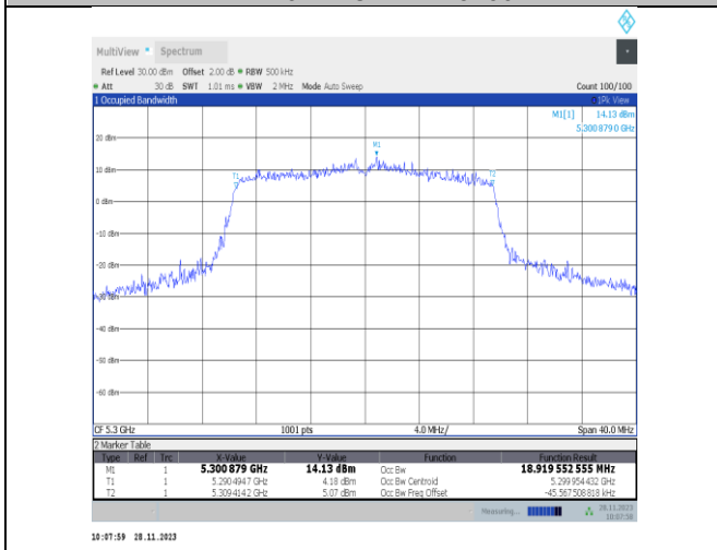
11ax20MIMO-Ant22-5300
