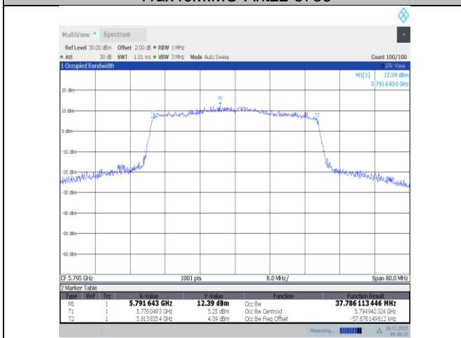
11ax40MIMO-Ant22-5795
