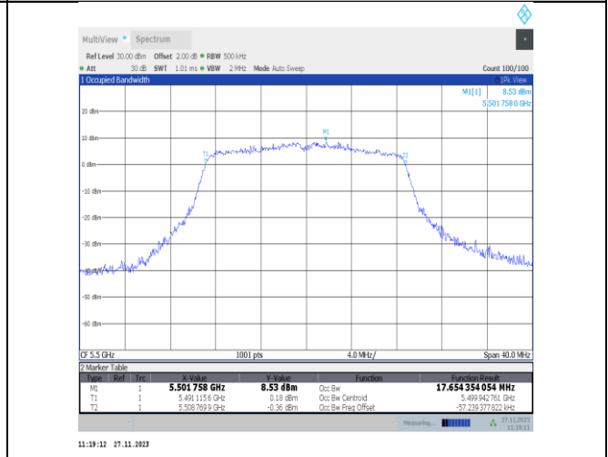
11n20MIMO-Ant25-5500
