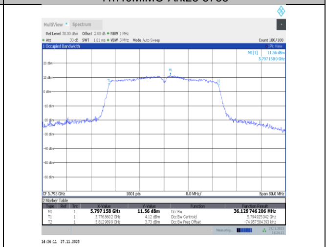
11n40MIMO-Ant25-5795
