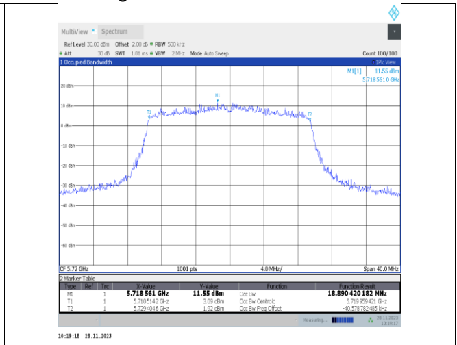
11ax20MIMO-Ant25-5720
