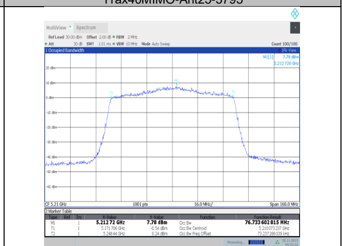
11ax80MIMO-Ant25-5210
