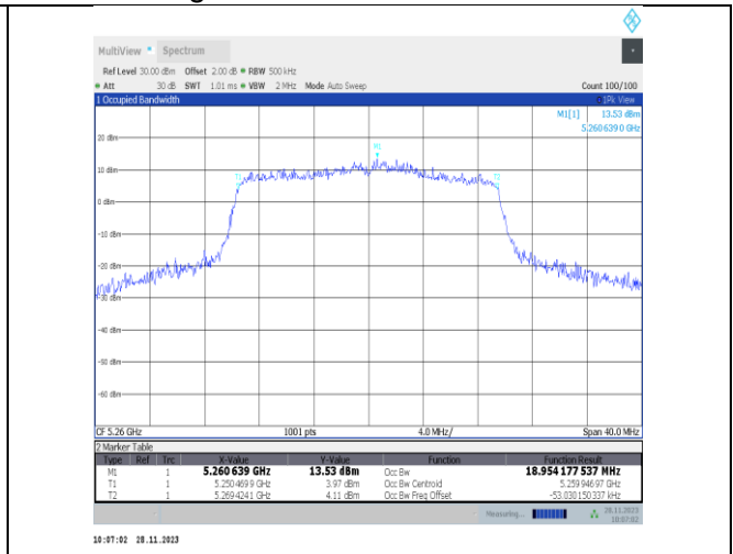
11ax20MIMO-Ant25-5260
