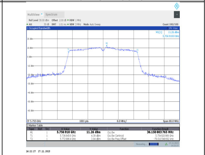
11n40MIMO-Ant25-5755
