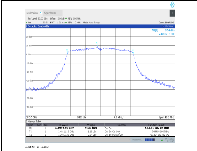
11n20MIMO-Ant22-5500
