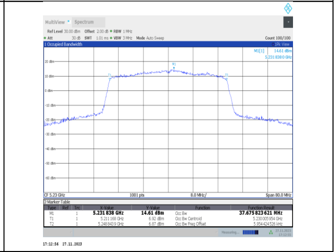
11ax40MIMO-Ant25-5230
