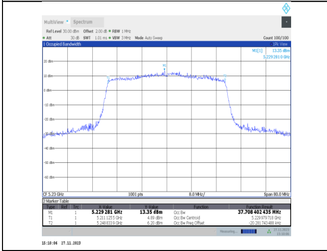
11ax40MIMO-Ant22-5230
