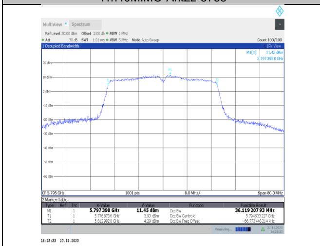
11n40MIMO-Ant22-5795
