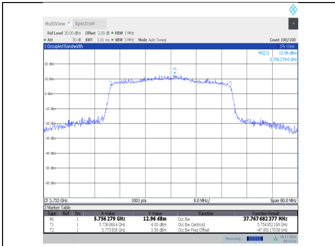
11ax40MIMO-Ant22-5755
