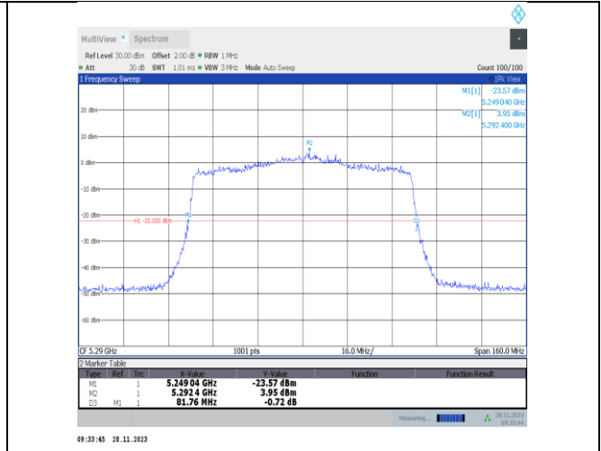
11ax80MIMO-Ant25-5290
