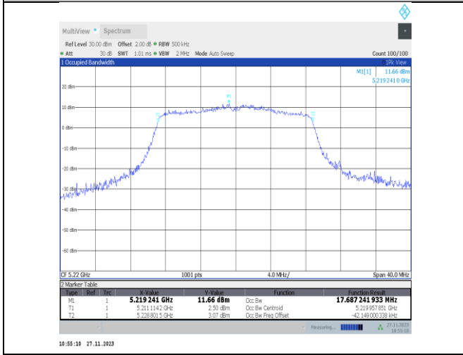
11n20MIMO-Ant22-5220
