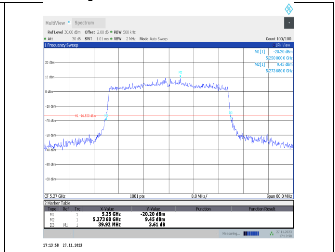
11ax40MIMO-Ant25-5270
