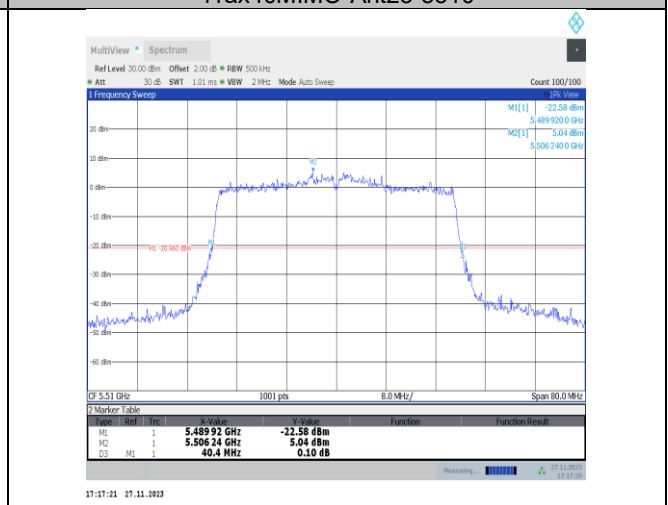
11ax40MIMO-Ant25-5510
