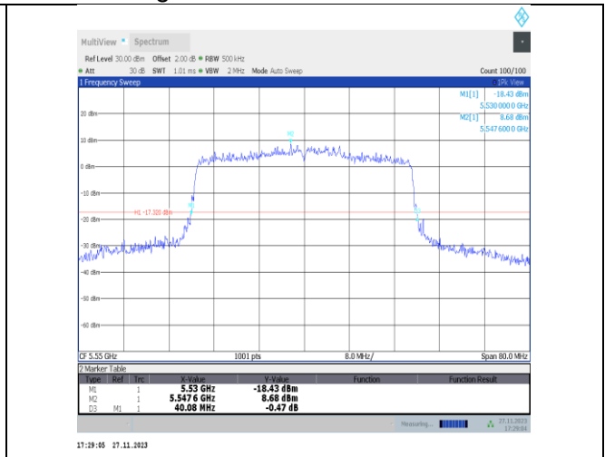
11ax40MIMO-Ant25-5550
