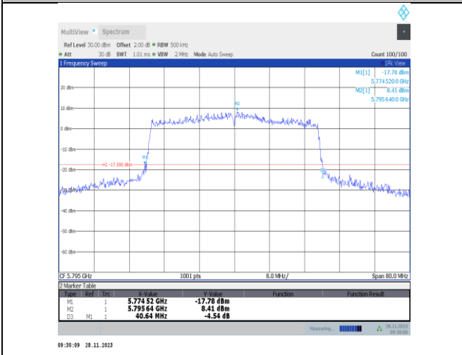
11ax40MIMO-Ant22-5795
