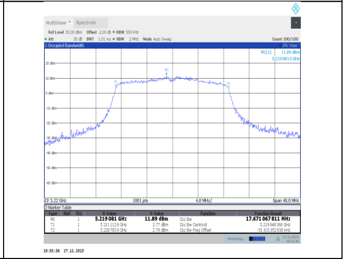
11n20MIMO-Ant25-5220
