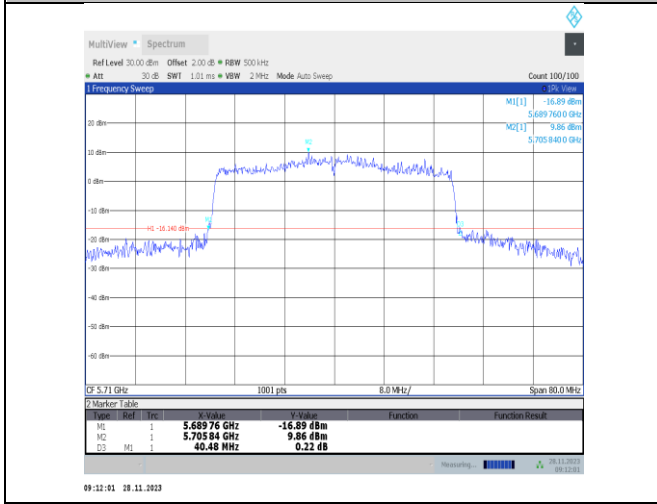
11ax40MIMO-Ant22-5710
