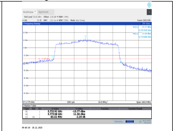
11ax80MIMO-Ant25-5775
