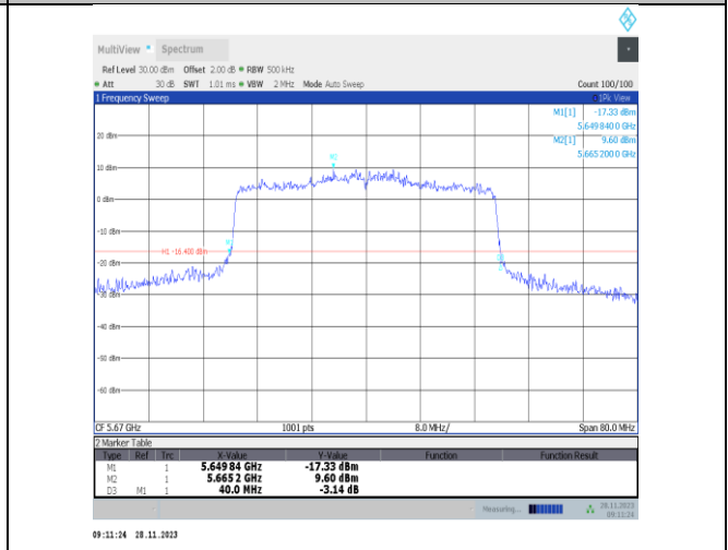
11ax40MIMO-Ant25-5670
