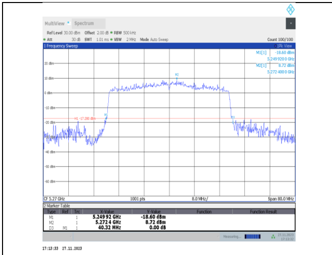
11ax40MIMO-Ant22-5270
