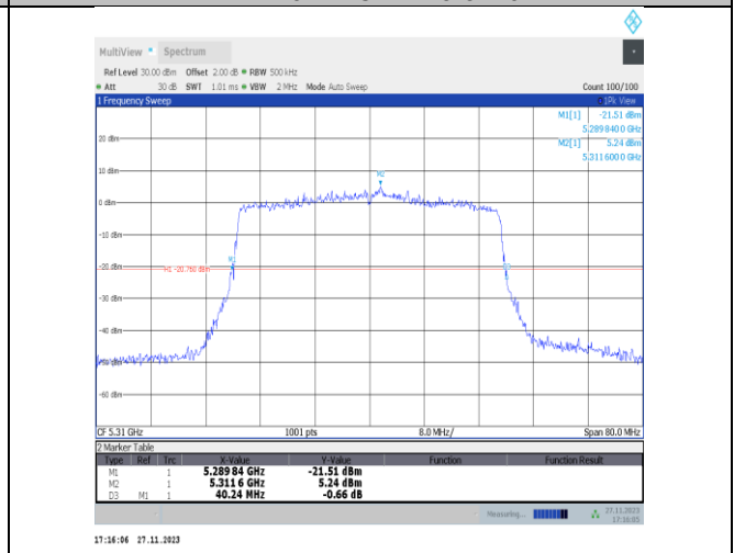
11ax40MIMO-Ant25-5310
