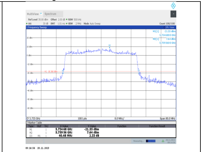
11ax40MIMO-Ant25-5755
