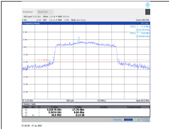
11ax40MIMO-Ant22-5550
