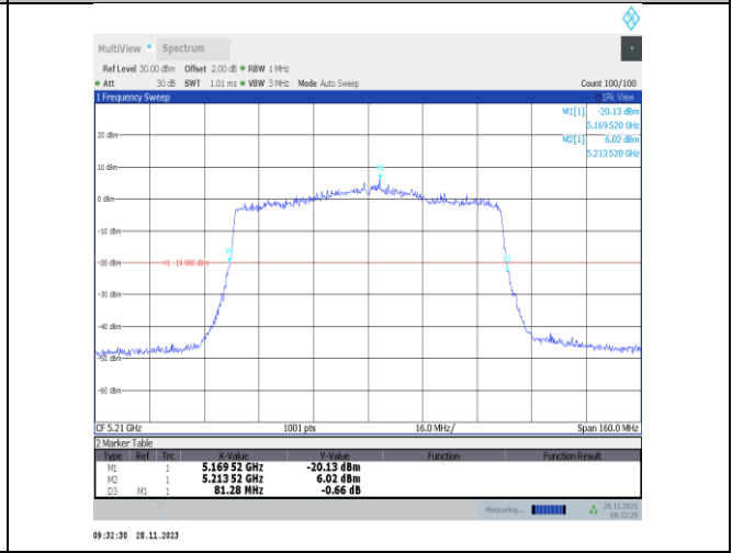
11ax80MIMO-Ant25-5210
