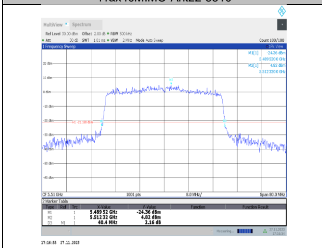
11ax40MIMO-Ant22-5510
