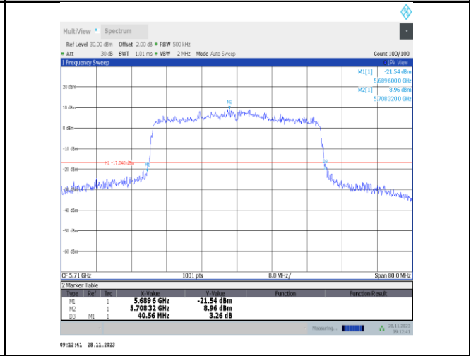
11ax40MIMO-Ant25-5710
