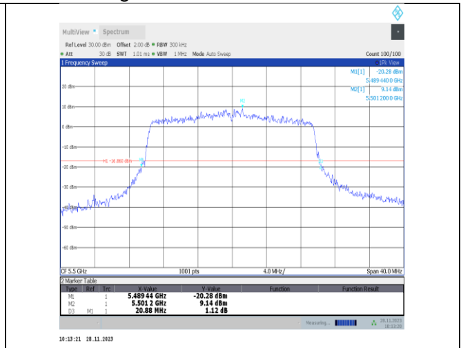
11ax20MIMO-Ant25-5500
