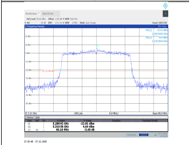
11ax40MIMO-Ant22-5310
