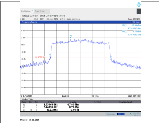
11ax40MIMO-Ant22-5755
