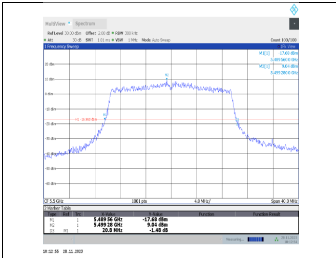
11ax20MIMO-Ant22-5500
