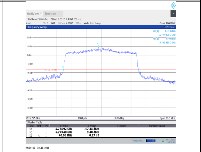
11ax40MIMO-Ant25-5795
