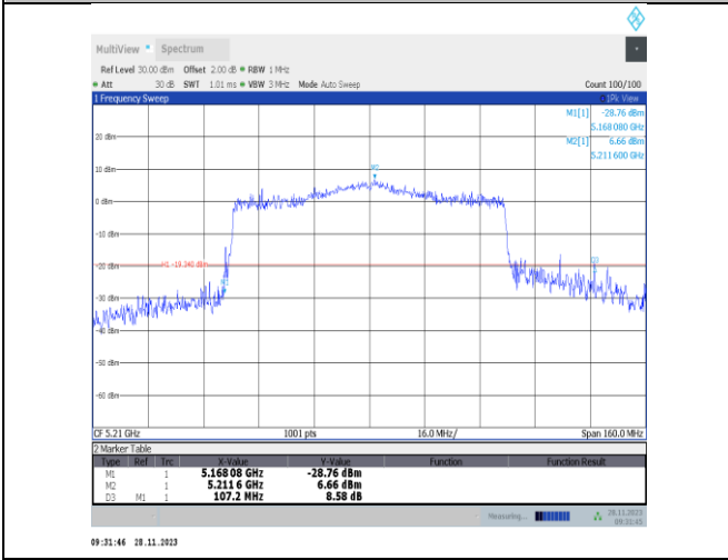
11ax80MIMO-Ant22-5210
