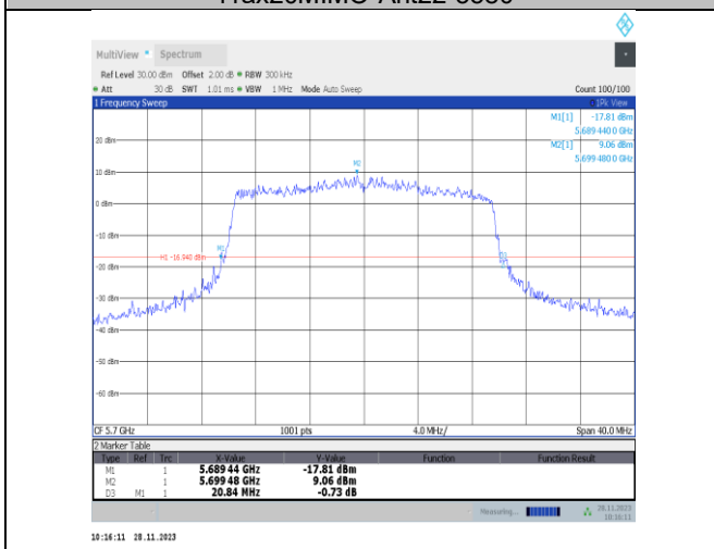
11ax20MIMO-Ant22-5700
