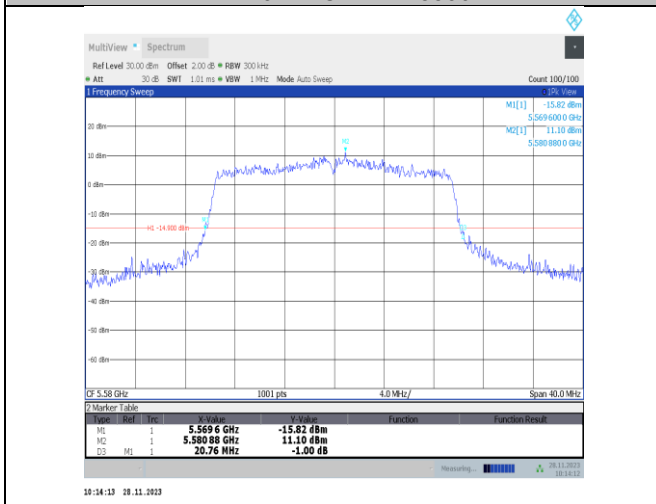
11ax20MIMO-Ant22-5580
