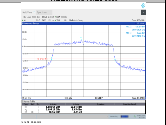
11ax20MIMO-Ant25-5700
