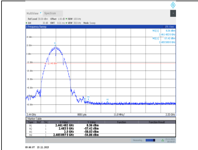
11b-CDD-Ant22-2462-PASS
