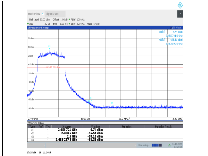
11ax20MIMO-Ant25-2457-PASS
