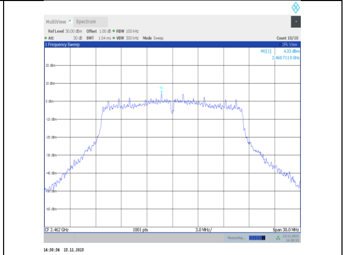
11g-CDD-Ant25-2462-0~Reference-PASS
