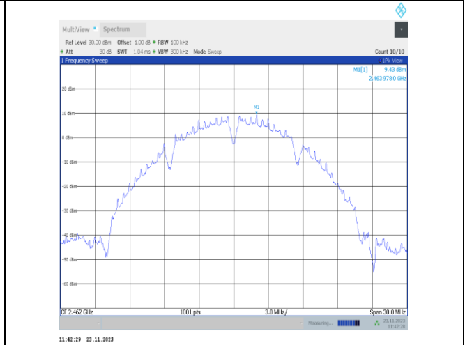
11b-CDD-Ant25-2462-0~Reference-PASS
