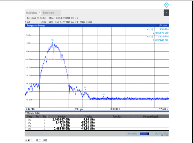
11b-CDD-Ant25-2462-PASS
