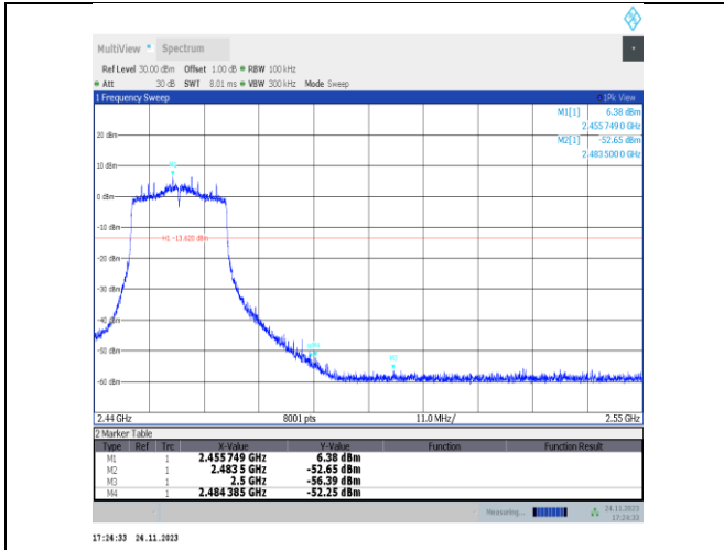
11ax20MIMO-Ant22-2457-PASS
