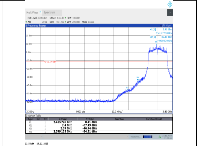
11g-CDD-Ant25-2417-PASS
