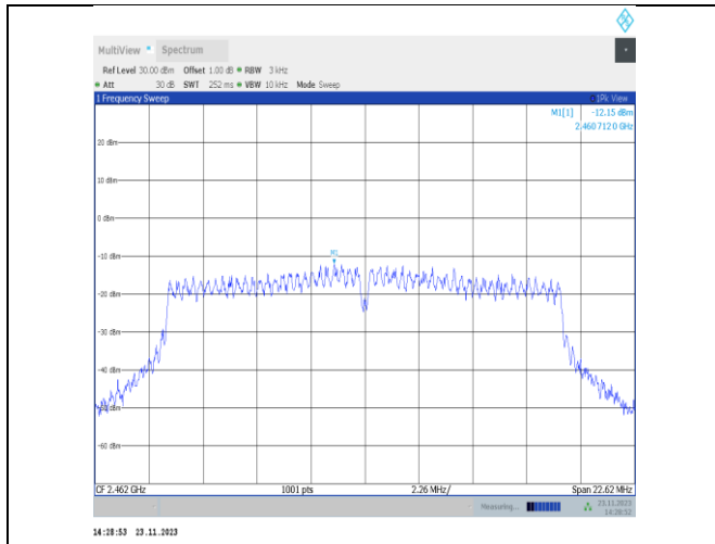
11g-CDD-Ant22-2462-PASS
