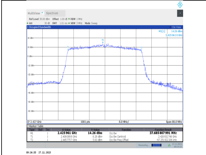
11ax40MIMO-Ant22-2427
