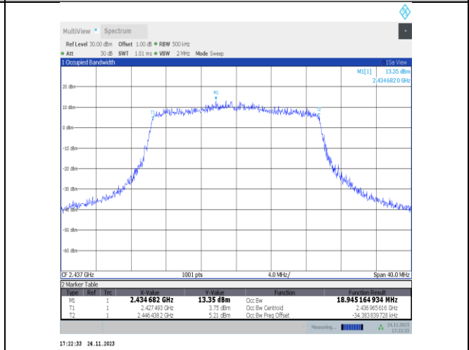
11ax20MIMO-Ant25-2437
