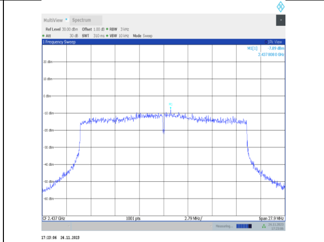
11ax20MIMO-Ant25-2437-PASS
