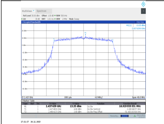
11ax20MIMO-Ant22-2437
