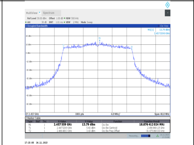
11ax20MIMO-Ant25-2457
