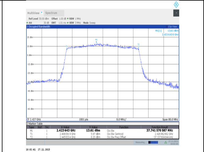
11ax40MIMO-Ant25-2427
