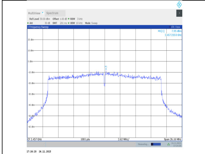
11ax20MIMO-Ant22-2457-PASS
