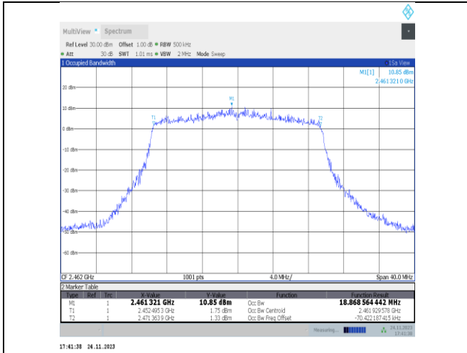
11ax20MIMO-Ant22-2462
