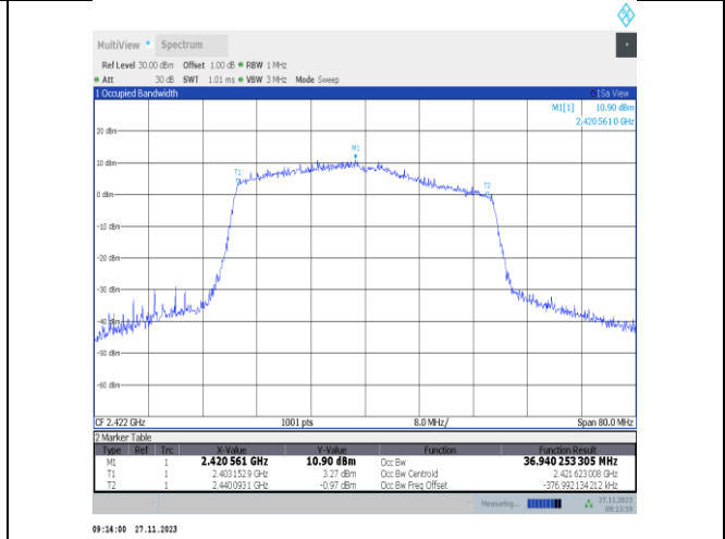
11ax40MIMO-Ant25-2422
