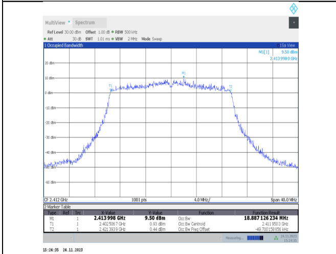
11ax20MIMO-Ant22-2412
