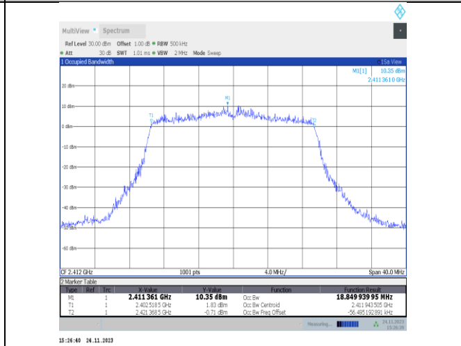
11ax20MIMO-Ant25-2412
