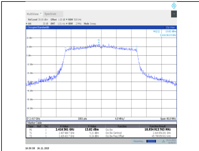
11ax20MIMO-Ant22-2417
