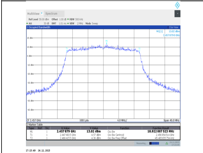
11ax20MIMO-Ant22-2457
