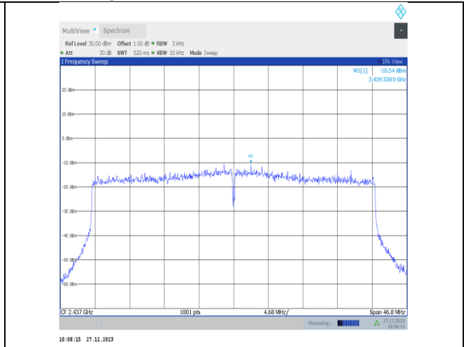
11ax40MIMO-Ant25-2437-PASS
