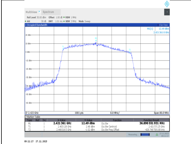
11ax40MIMO-Ant22-2422
