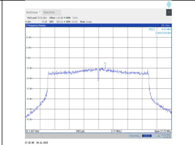
11ax20MIMO-Ant25-2457-PASS
