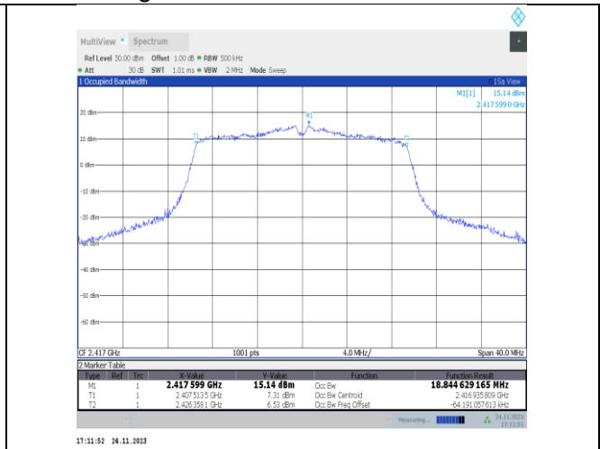
11ax20MIMO-Ant25-2417
