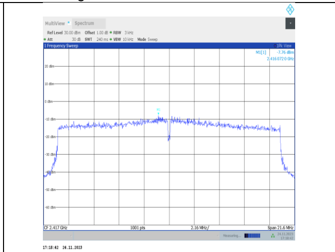
11ax20MIMO-Ant25-2417-PASS
