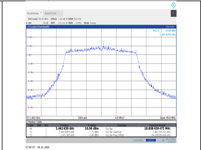
11ax20MIMO-Ant25-2462
