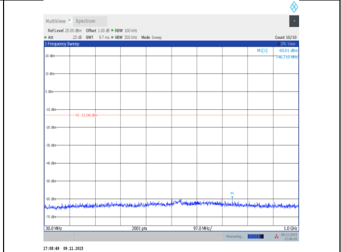
BLE_2M-Ant25-2440-30~1000-PASS
