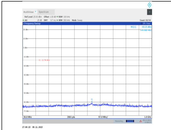
BLE_2M-Ant25-2402-30~1000-PASS
