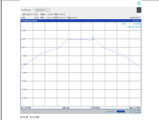
DH5-Ant25-2480-0~Reference-PASS
