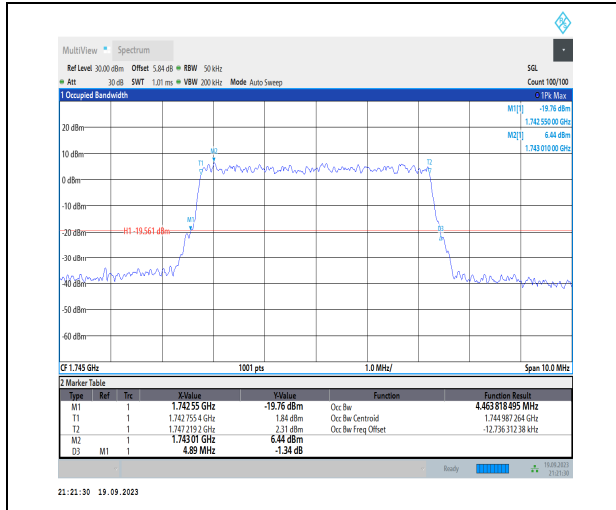
1-N66-PC3-15-5-M-9-CP-256QAM-Outer_Full-25@0 -Ant31-4.464-4.890-≤5-PASS
