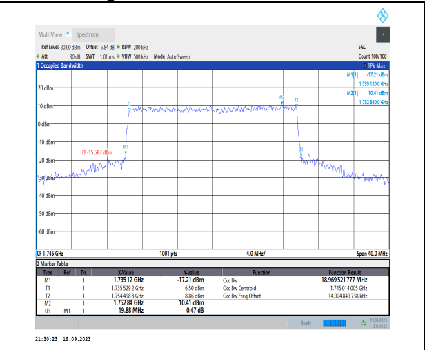
1-N66-PC3-15-20-M-7-CP-16QAM-Outer_Full-106@0 0-Ant31-18.97-19.880-≤20-PASS
