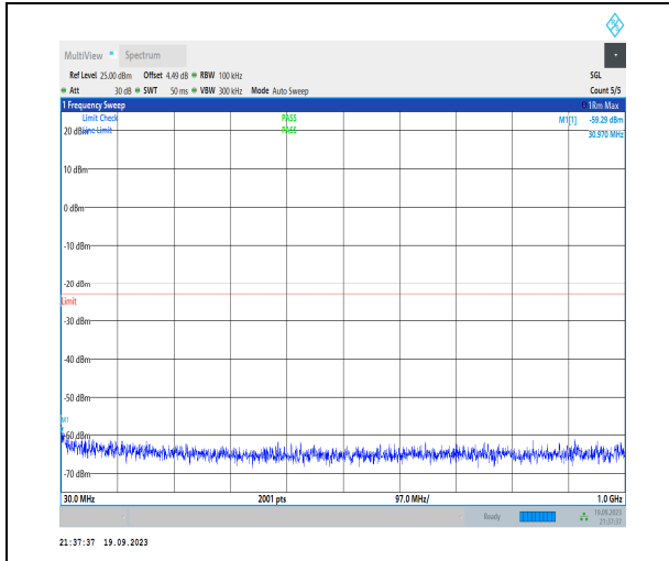
1-N66-PC3-15-40-M-1-DFT-PI2BPSK-Inner_1RB_L eft-1@1-30-1000-Ant31-30.97--59.29--23-PASS
