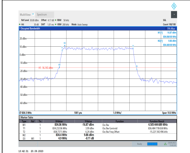
1-N26-824-849-PC3-15-5-M-7-CP-16QAM-Outer_Fu. II-25@0-Ant41-4.505-4.900-≤5-PASS
