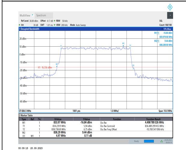
1-N5-PC3-15-5-M-7-CP-16QAM-Outer_Full-25@0-A nt41-4.499-4.970-≤5-PASS
