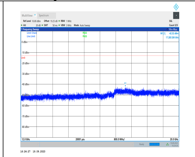
1-N2-PC3-15-20-L-1-N/A-DFT-PI2BPSK-Inner_1RB_ Left-1@1-12000-20000-Ant31-17283.20--42.32--13-P ASS
