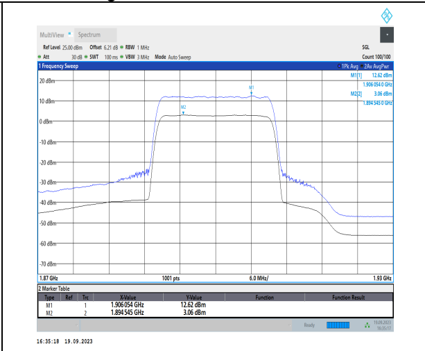
1-N2-PC3-15-20-H-2-CP-256QAM-Outer_Full-106@ 0-Ant31-9.56-100%-0.00-9.56-PASS<13
