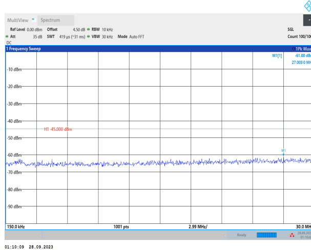
Band7-20MHz-QPSK-20850-1RB#0-Range2:0.15~30MHz
