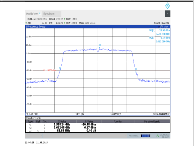
11ac80SISO-Ant23-5610
