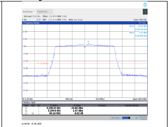
11ac80SISO-Ant23-5290
