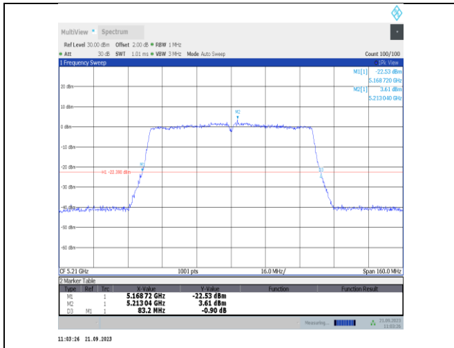
11ac80SISO-Ant23-5210
