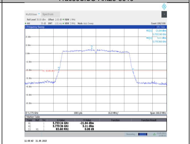
11ac80SISO-Ant23-5775
