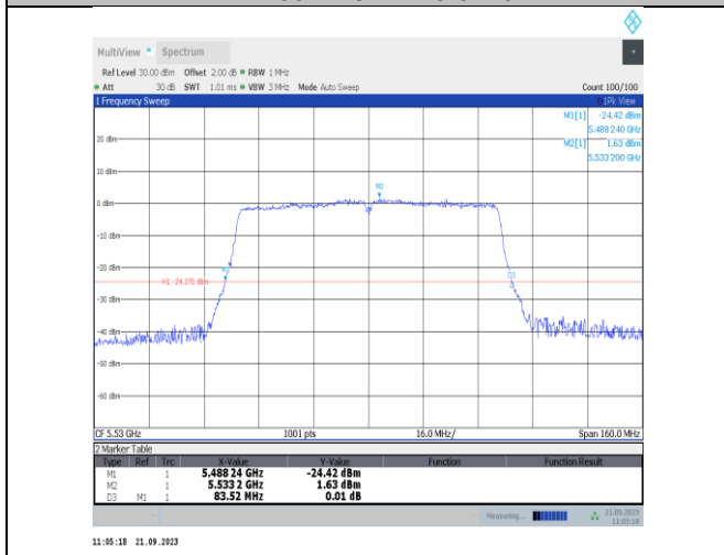
11ac80SISO-Ant23-5530
