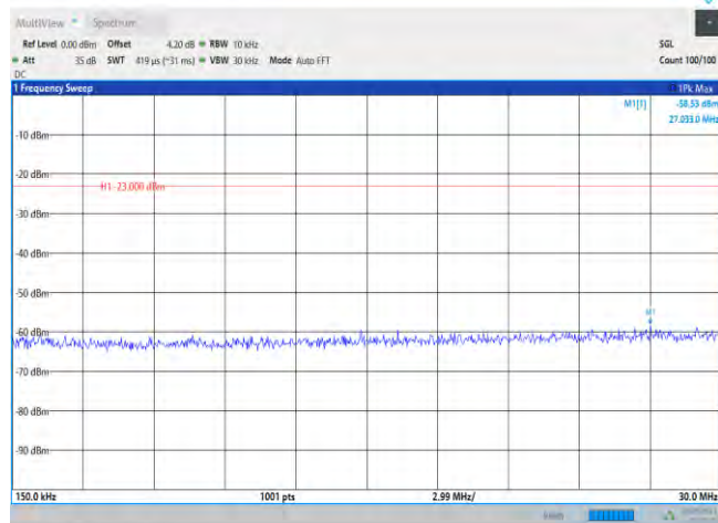
Band12-10MHz-QPSK-23060-1RB#0-Range2:0.15~30MHz
