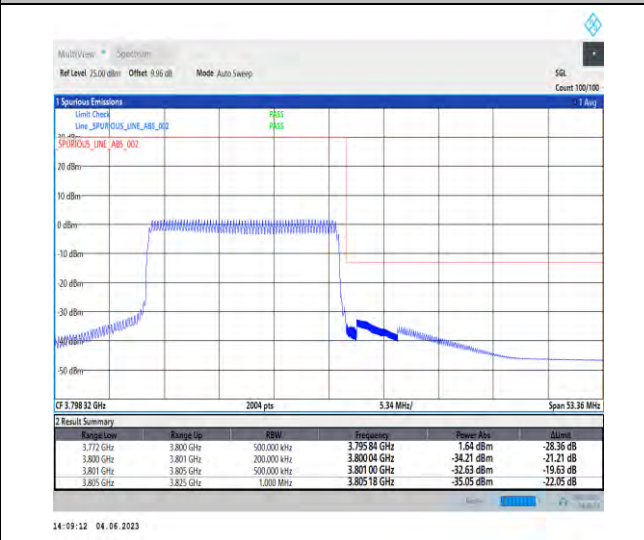
NTNV_N78-3700-3800_PC2_30_20_H_TID6_RID1#1
