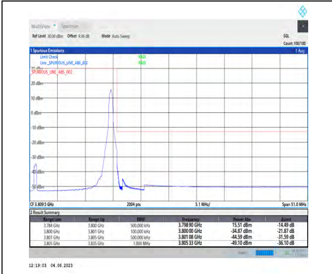
NTNV_N78-3700-3800_PC2_30_30_H_TID2_RID1#1
