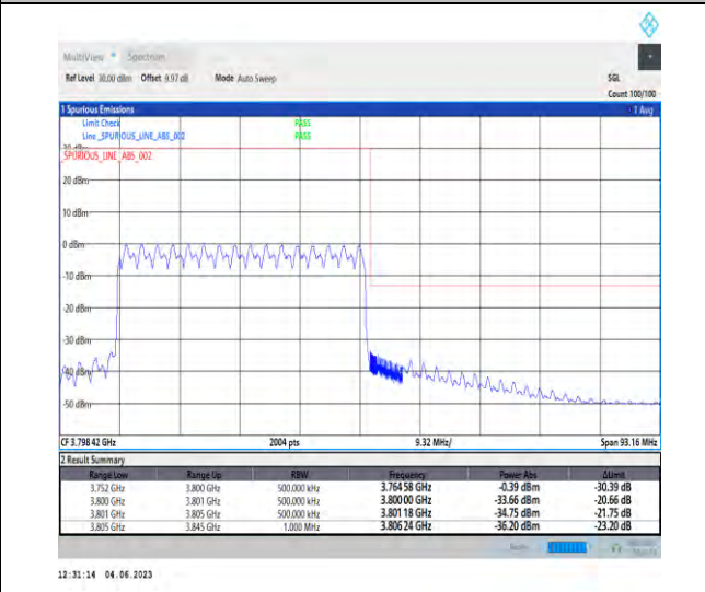
NTNV_N78-3700-3800_PC2_30_40_H_TID6_RID1#1
