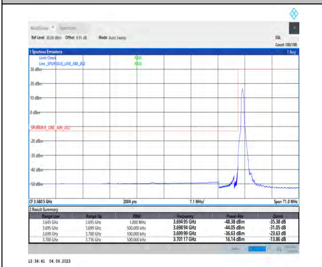
NTNV_N78-3700-3800_PC2_30_50_L_TID4_RID1#1
