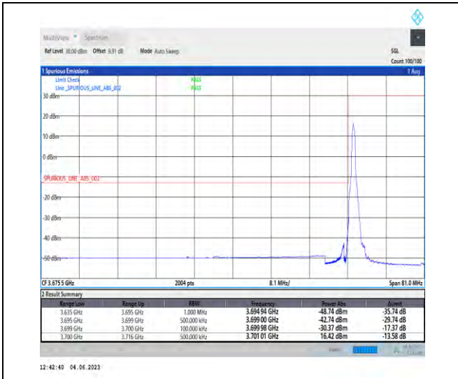
NTNV_N78-3700-3800_PC2_30_60_L_TID1_RID1#1
