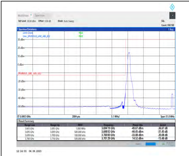
NTNV_N78-3700-3800_PC2_30_30_L_TID1_RID1#1
