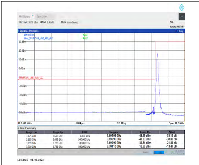
NTNV_N78-3700-3800_PC2_30_70_L_TID1_RID1#1
