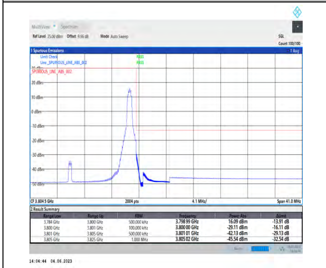
NTNV_N78-3700-3800_PC2_30_20_H_TID5_RID1#1
