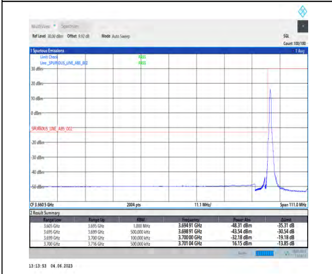
NTNV_N78-3700-3800_PC2_30_90_L_TID4_RID1#1
