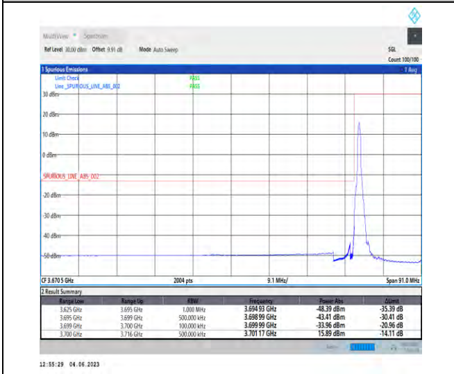
NTNV_N78-3700-3800_PC2_30_70_L_TID4_RID1#1
