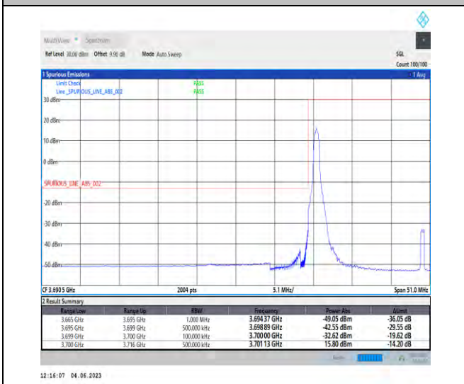
NTNV_N78-3700-3800_PC2_30_30_L_TID4_RID1#1
