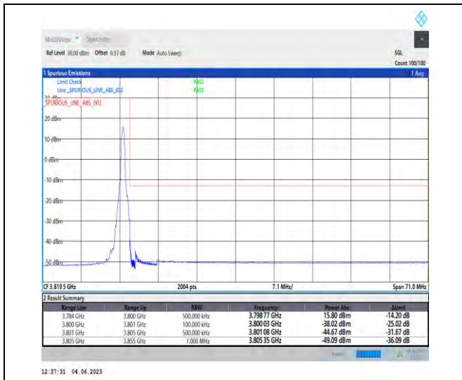
NTNV_N78-3700-3800_PC2_30_50_H_TID2_RID1#1
