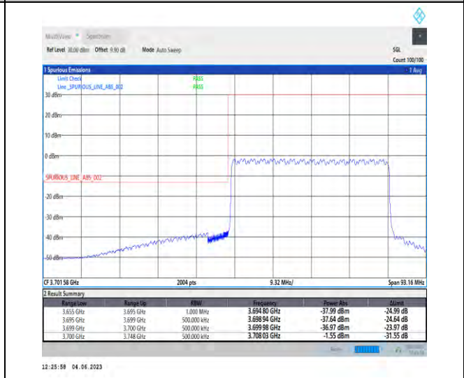
NTNV_N78-3700-3800_PC2_30_40_L_TID6_RID1#1
