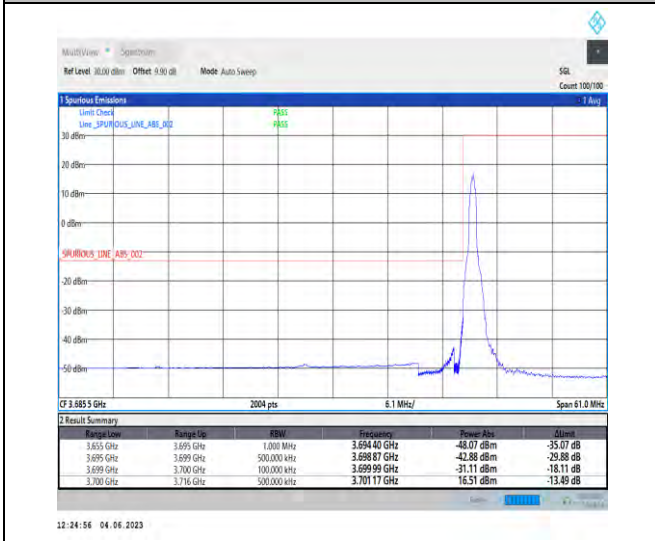
NTNV_N78-3700-3800_PC2_30_40_L_TID4_RID1#1
