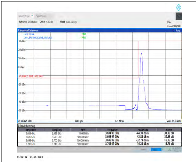
NTNV_N78-3700-3800_PC2_30_40_L_TID1_RID1#1
