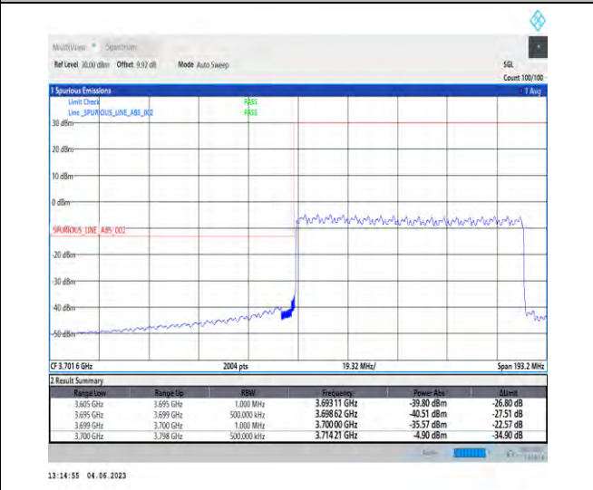
NTNV_N78-3700-3800_PC2_30_90_L_TID6_RID1#1
