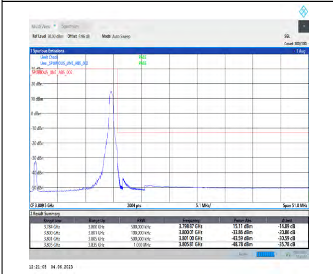
NTNV_N78-3700-3800_PC2_30_30_H_TID5_RID1#1
