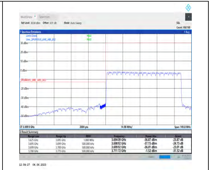
NTNV_N78-3700-3800_PC2_30_70_L_TID3_RID1#1
