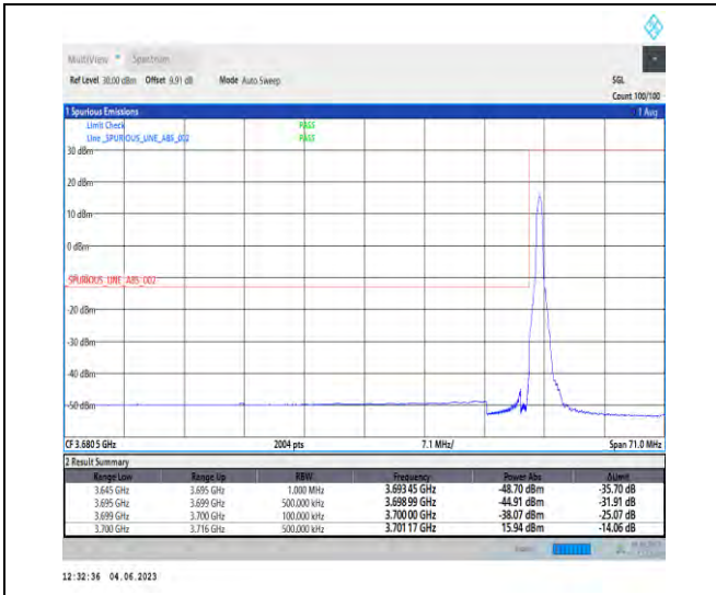
NTNV_N78-3700-3800_PC2_30_50_L_TID1_RID1#1
