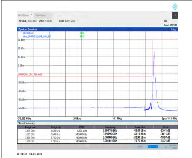
NTNV_N78-3700-3800_PC2_30_80_L_TID4_RID1#1
