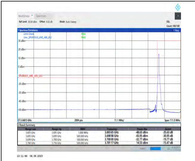
NTNV_N78-3700-3800_PC2_30_90_L_TID1_RID1#1
