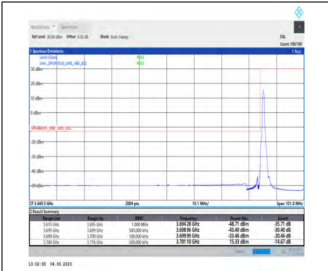
NTNV_N78-3700-3800_PC2_30_80_L_TID1_RID1#1
