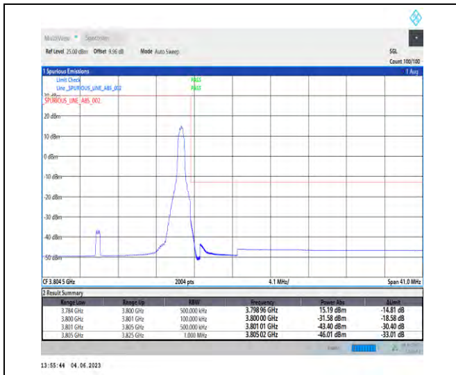
NTNV_N78-3700-3800_PC2_30_20_H_TID2_RID1#1
