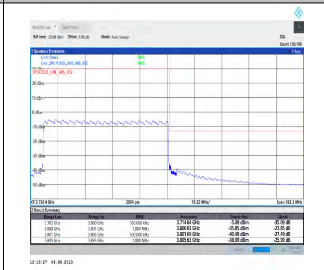
NTNV_N78-3700-3800_PC2_30_90_H_TID6_RID1#1
