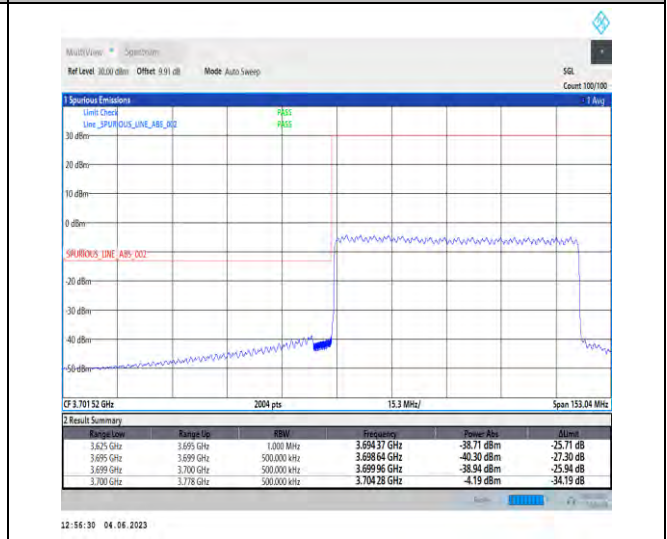
NTNV_N78-3700-3800_PC2_30_70_L_TID6_RID1#1
