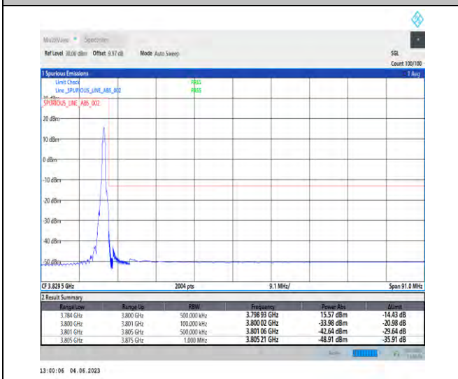
NTNV_N78-3700-3800_PC2_30_70_H_TID5_RID1#1
