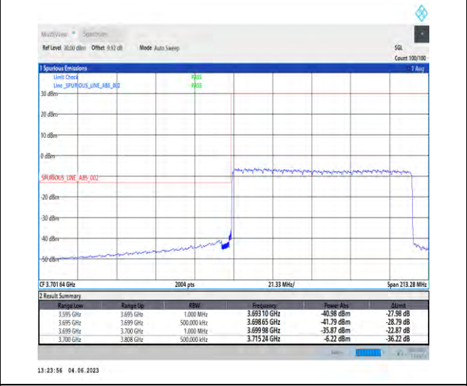
NTNV_N78-3700-3800_PC2_30_100_L_TID6_RID1#1
