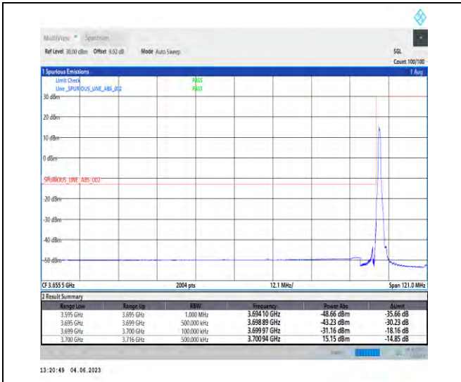
NTNV_N78-3700-3800_PC2_30_100_L_TID1_RID1#1
