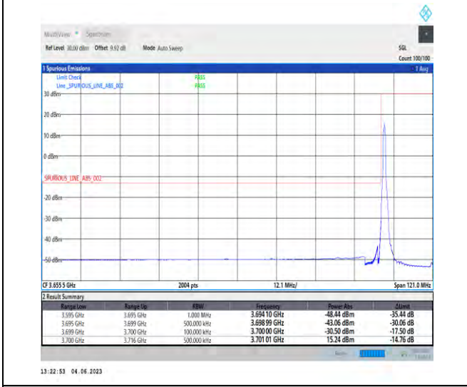
NTNV_N78-3700-3800_PC2_30_100_L_TID4_RID1#1
