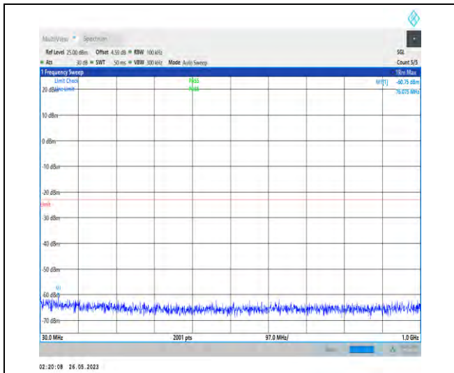
1-N66-PC3-15-40-M-1-DFT-PI2BPSK-Inner_1RB_L eft-1@1-30-1000-34.85--59.79--23-PASS
