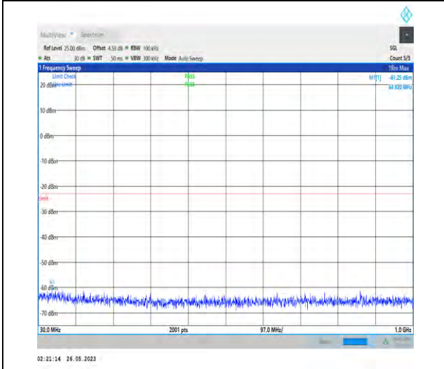
1-N66-PC3-15-40-H-1-DFT-PI2BPSK-Inner_1RB_L eft-1@1-30-1000-32.91--59.44--23-PASS
