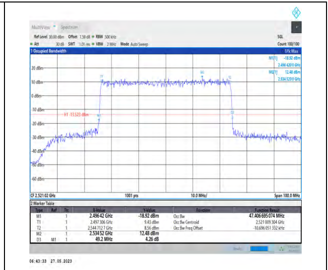
1-N41-PC3-30-50-L-6-CP-QPSK-Outer_Full-133@0 -47.407-49.200-≤50-PASS
